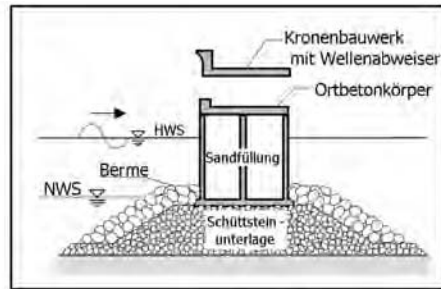
(b) zusammengesetzter Wellenbrecher
