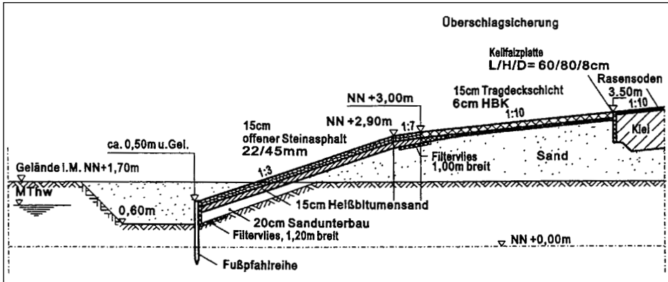
Abb. G 1a: Vorlanddeckwerk Friedrich-Wilhelm-Lübke-Koog
