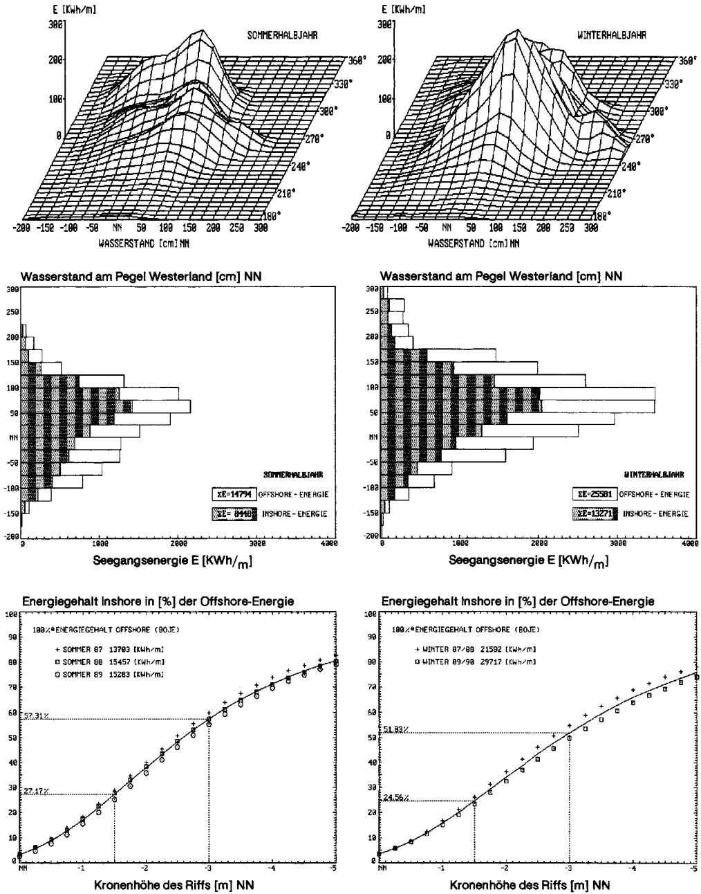
Abb. A 3.38: Vergleichende Darstellung der Offshore- und Inshore Wellenenergien und Einfluss der Kronenhöhe des Riffs, Beispiel Sylt (STROTMANN u. KOHLHASE, 1991)
