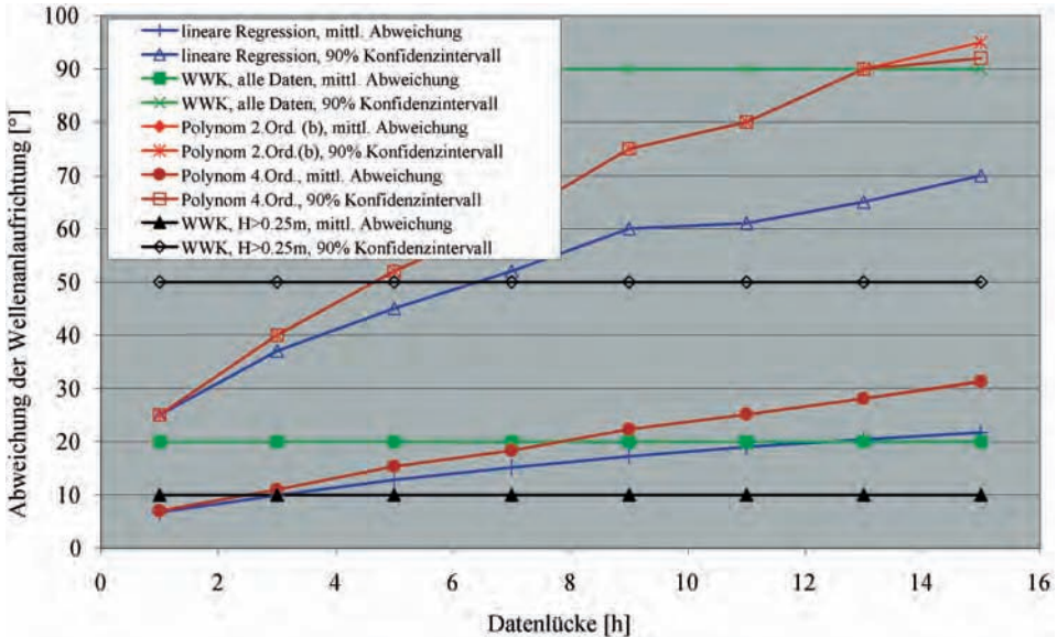
Abb. A 3.53: Abweichung von berechneten Wellenanaufrichtungen von Messwerten für ausgewählte Verfahren zur Schließung von Datenlücken
