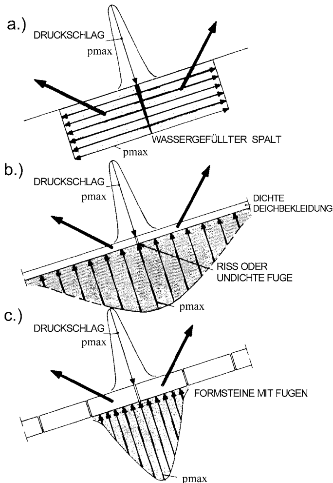
Abb. A 4.2.6: Sprengwirkungen von Druckschlägen auf Risse und Fugen (nach FÜHRBÖTER, 1966)
