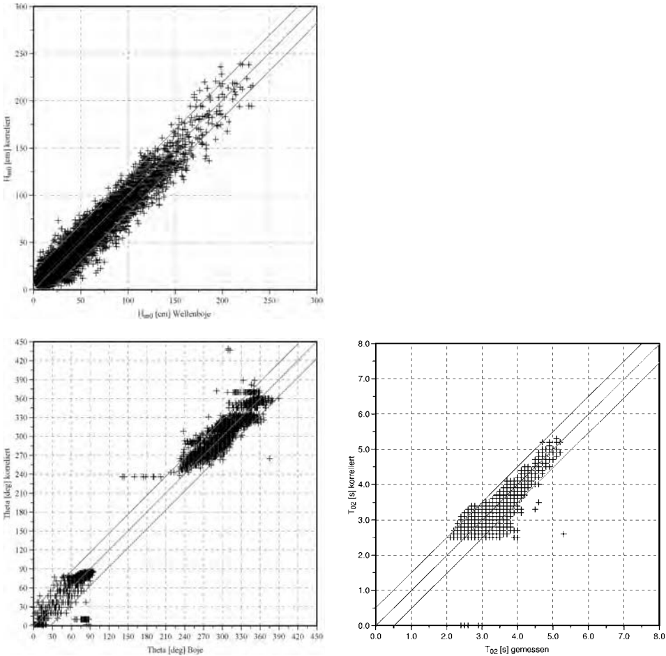
Abb. A 3.50: Berechnete und gemessene Seegangparameter mit linearer Regression und 90 % Konfidenzintervallen (FRÖHLE et al., 1999)
