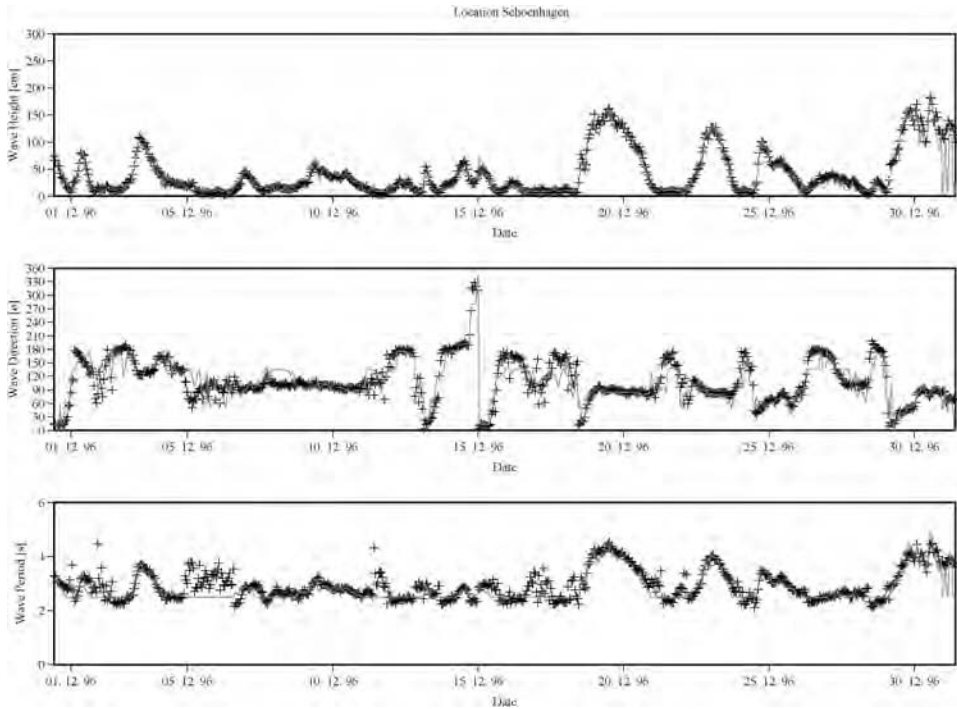
Abb. A 3.51: Gemessene (+) und berechnete (—) Wellenparameter. Projektgebiet Heiligenhafen (vgl. FRÖHLE et al., 1997)
