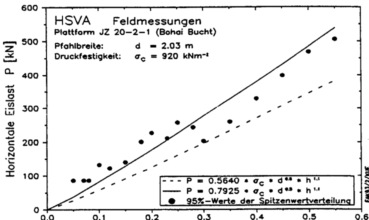
Abb. A 7.12: Horizontale Eislast als Funktion der Eisdicke am Bauwerk JZ 20-2-1 in der Bohai-Bucht
