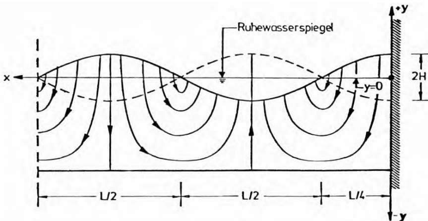
Abb. A 5.9: Schematisches Stromlinienbild einer stehenden Welle
