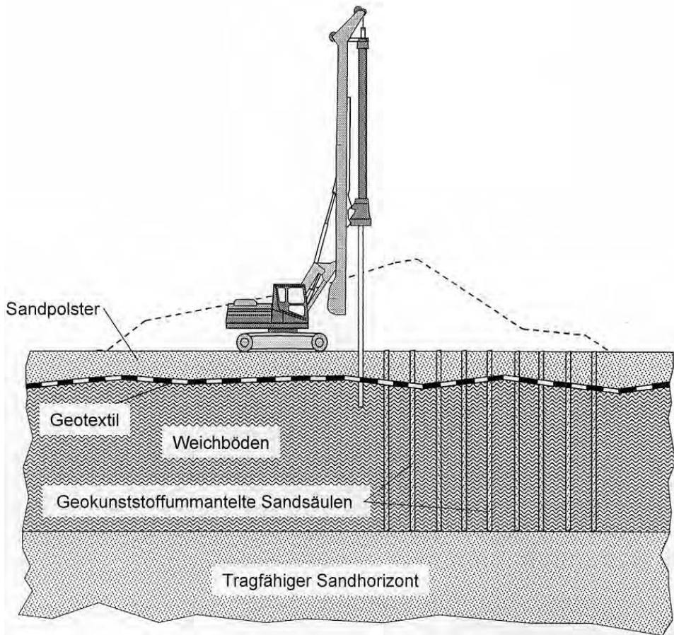
Abb. G 42: Gründungssystem aus Geokunststoff bewehrten Tragschichten und geokunststoffummantelte Sandsäulen
