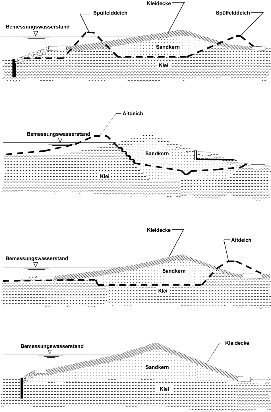
Abb. B 1: Bodenaufbau von Deichprofilen an der Nordseeküste
