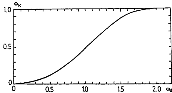
Abb. A 3.14: Verlauf von \Phi_K in Abhängigkeit von \omega_d (nach KITAIGORODSKII et al., 1975)
