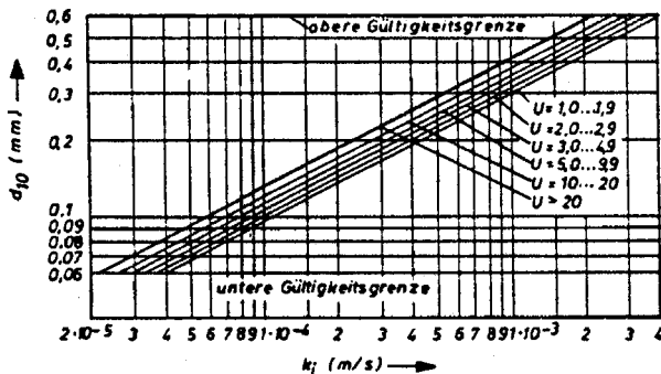
Abb. 1. Beziehung zwischen d_{10} und der DurchlÄssigkeit k in AbhÄngigkeit von U nach BEYER (WWT, H. 6, S. 165, 1964)
