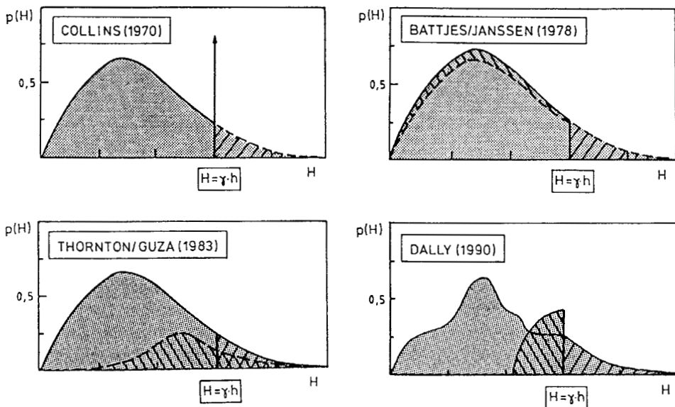
Abb. A 3.25: Zur Ermittlung des Anteils brechender Wellen (OELERICH, 1990)
