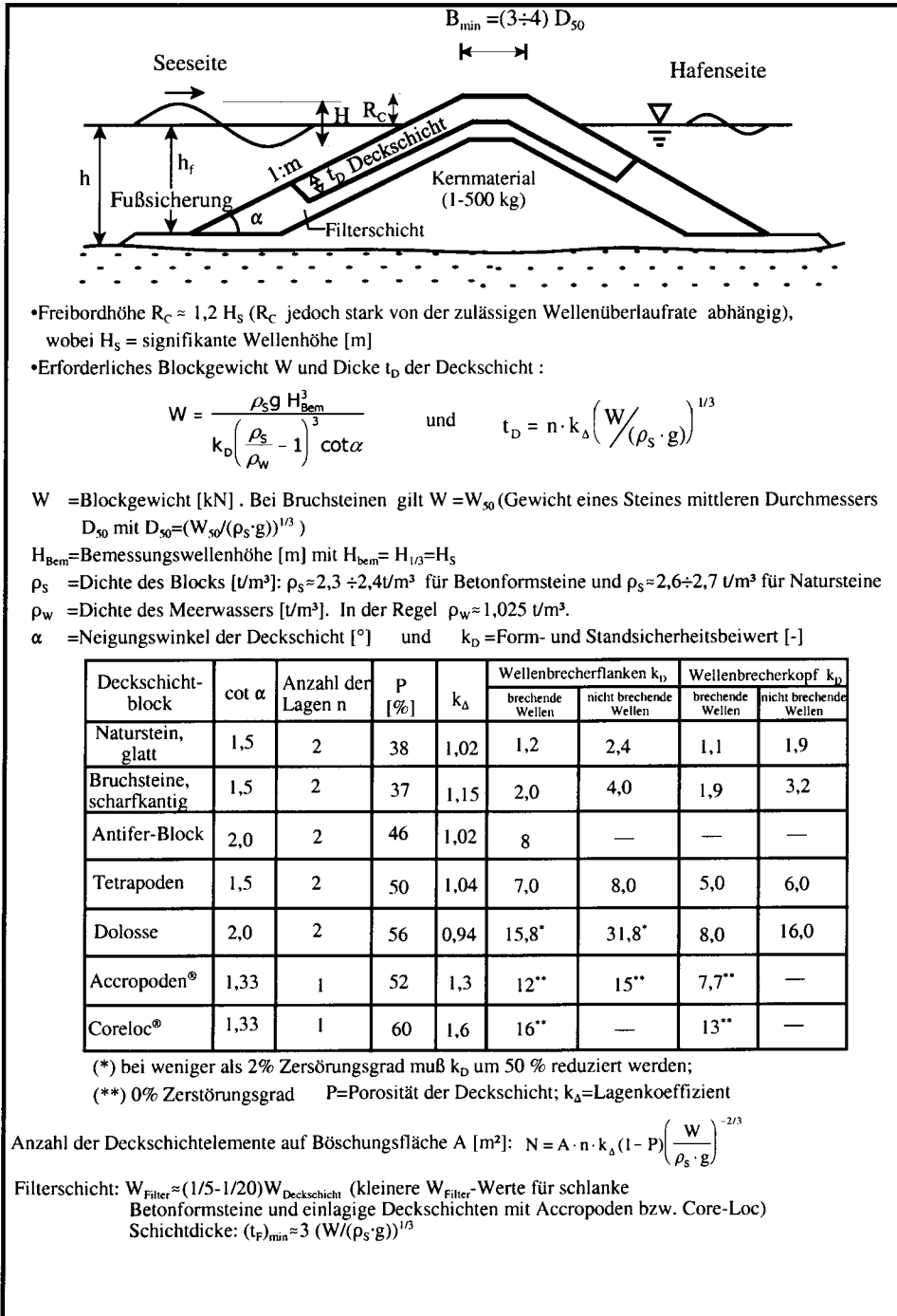
Abb. A 4.2.14: Bemessungsformeln für geschüttete Wellenbrecher – HUDSON-Formel (OUMERACI, 2001)
