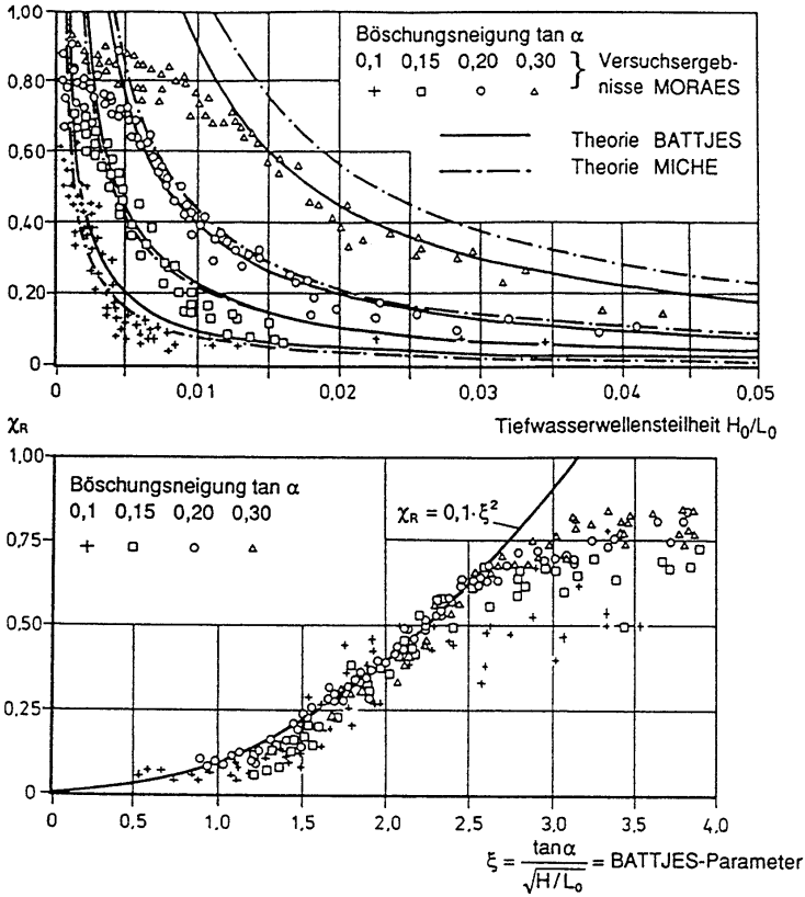
Abb. A 3.29: Reflexion an glatten Böschungen (BATTJES, 1974)
