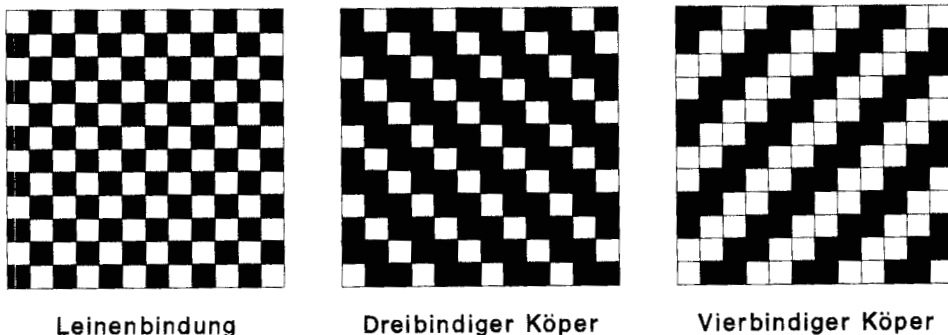
Abb. C 8: Bindungspatronen von Geweben (SAATHOFF u. ZITSCHER, 2001)
