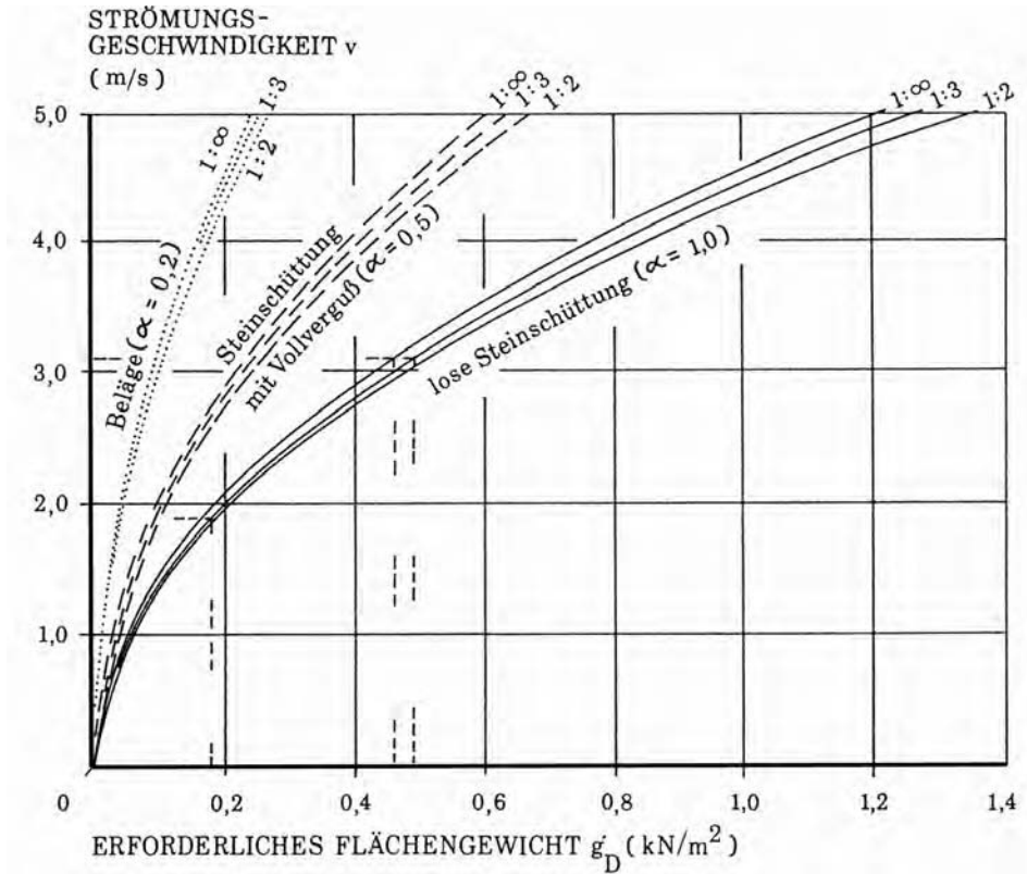
Abb. A 5.11: Erforderliches Flächengewicht von gebundenen Böschungs- und Sohlauskleidungen (durchlässig bei einer Stabilität gegen Abheben von n_z = 1,2 in Abhängigkeit von der Überströmung [bei Schublagerung])
