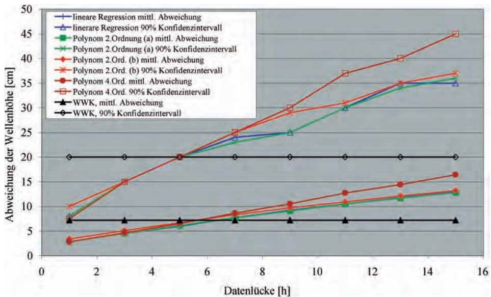
Abb. A 3.52: Abweichung von berechneten Wellenhöhen von Messwerten für ausgewählte Verfahren zur Schließung von Datenlücken
