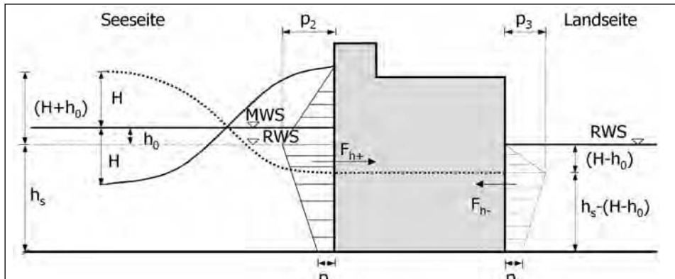
Tafel A 4.3.3: Druckbelastung durch stehende Wellen (Verfahren nach SAINFLOU und Hinweise auf das Verfahren von MICHE-RUNDGREN)
