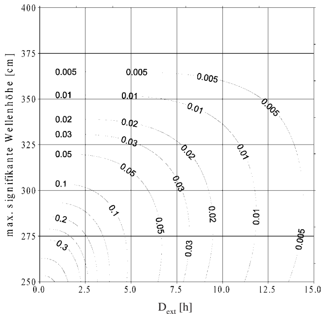
Abb. A 8.8: Gemeinsame Überschreitungswahrscheinlichkeit der Dauer ( D_{\text{ext}} ) und der maximalen signifikanten Wellenhöhe ( H_{m0,\text{max}} ) innerhalb eines Extremereignisses (Daten Heiligenhafen, Ostsee) (Kombinierte univariate Methode, Vergleichswellenhöhe für die Berechnung der Dauer H_{m0,\text{vgl}} = 2,46 \hat{=} 1 -jährliche Wellenhöhe)
