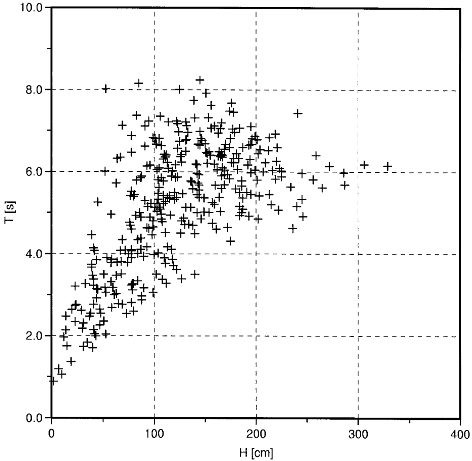
Abb. A 3.9: Punktediagramm der Wellenhöhen und Perioden einer Auswertung im Zeitbereich
