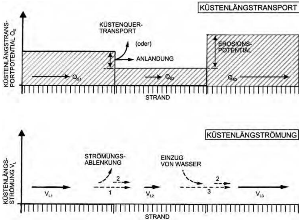
Abb. A 6.9: Schematische Verteilung des Transportpotentials entlang einer Küste infolge Refraktion und Shooling sowie infolge veränderlichen Verlaufs der Küstenlinie. Die Küstenlängsströmung ist der küstenparallelen Komponente des Energieflusses sowie dem Küstenlängstransportpotential proportional
