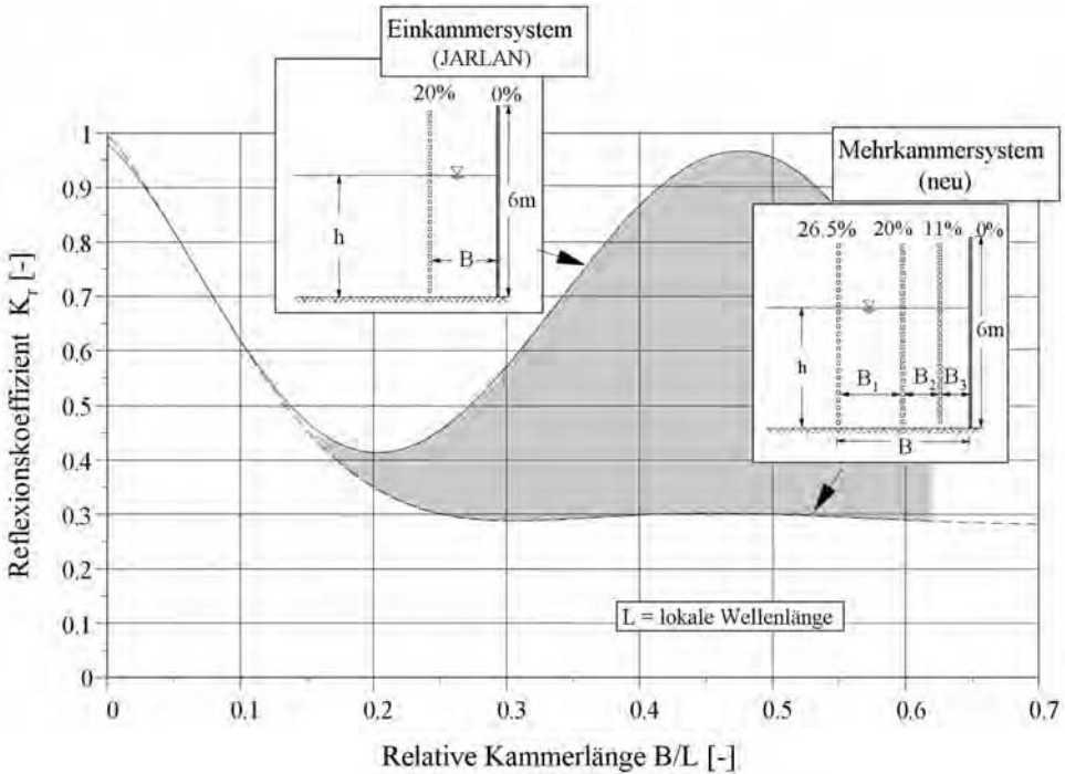
Abb. A 4.3.7: Funktionskurven eines vertikalen Bauwerks mit einer Wellenkammer (EKS) und für ein Mehrkammersystem (MKS)
