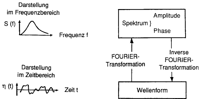
Abb. A 3.44: Zusammenhänge zwischen Frequenz- und Zeitbereichsdarstellung, schematisch
