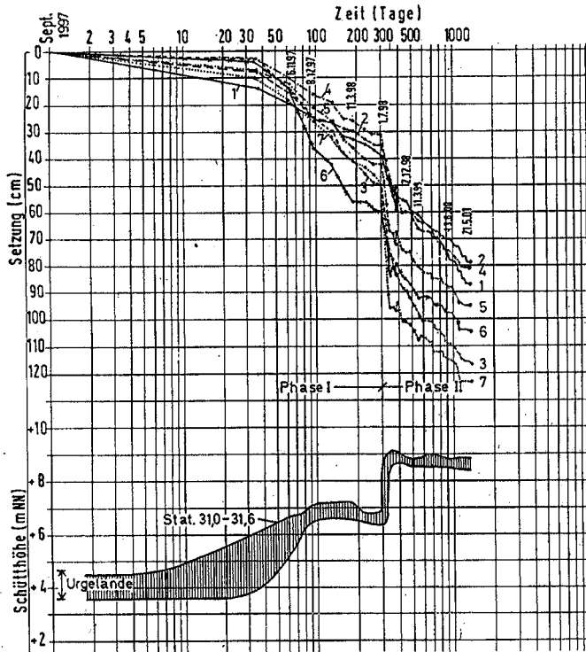
Abb. B 15: Setzungsmessungen verschiedener Stationen mit Prognose der Restsetzungen für den Verstärkungsabschnitt
