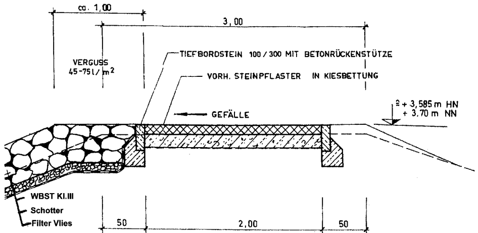
Abb. G 57 : Verklammertes Deckwerk mit Anschluss an die Spundwand im Hafen (Hiddensee)
