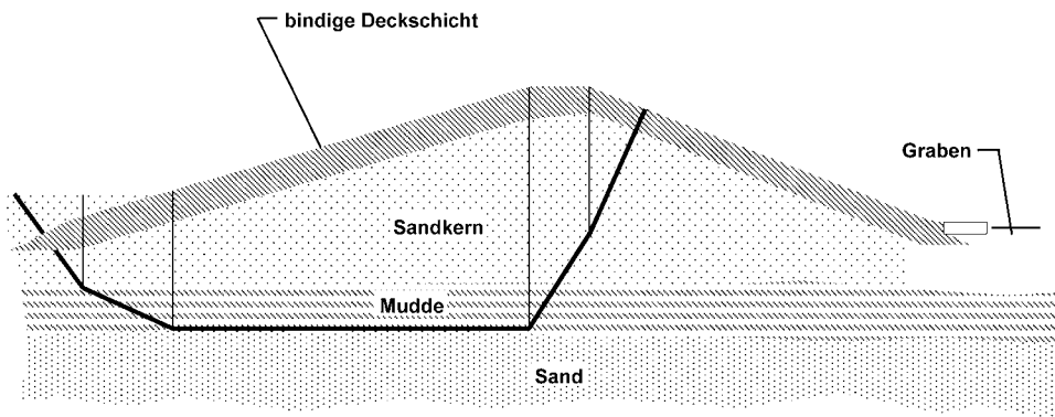
Abb. B 6: Beispiel einer Standsicherheitsuntersuchung nichtkreisförmiger Gleitkörper eines Ostseedeiches
