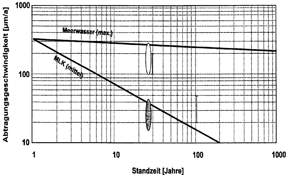
Abb. C 20: Mittlere bzw. maximale Abtragungsgeschwindigkeiten im Mittellandkanal (MLK) und Meerwasser nach (BINDER, 2001) Schwarzes Feld: Aktuelle Messungen „Unterwasserzone“; Eingerahmtes Feld: Aktuelle Messungen „Spritzwasserzone“; Balken: Berechnung nach DIN 50929
