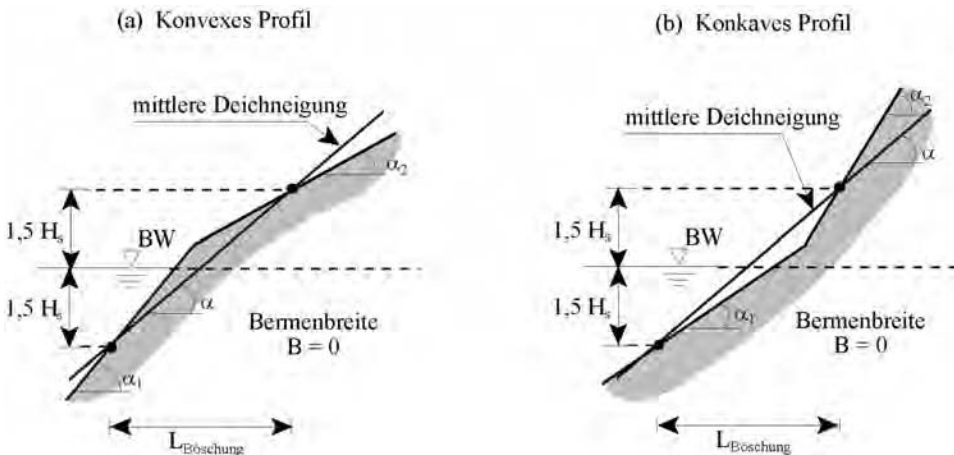
Abb. A 4.2.9: Definition der mittleren Deichneigung \alpha für ein konkaves und ein konvexes Deichprofil
