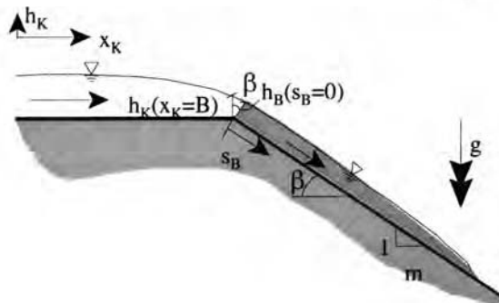
Abb. A 4.2.13: Definition der Strömungsgrößen auf Deichkrone und Deichbinnenböschung
