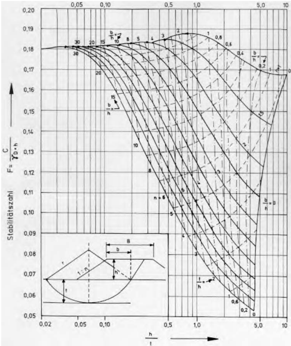
Abb. B 7: Standsicherheitsabschätzung für den Bauzustand nach SIEDEK, GRASSHOFF, KÜBLER (1969)
