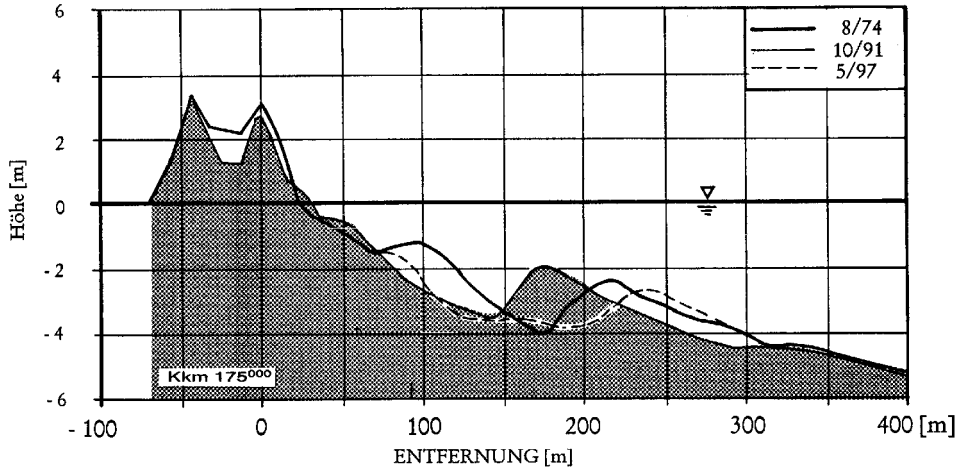
Abb. A 6.8: Überlagerung von Profilaufmaßen über einen Zeitraum von mehr als 20 Jahren (1974–1997) zur Veranschaulichung der aktiven Zone im Bereich der Fischlandküste (DETTE et al., 2001)
