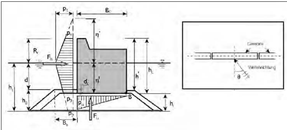
Tafel A 4.3.2: Verfahren von GODA für die Druckbelastung nichtbrechender, brechender und gebrochener Wellen (ohne Druckschlag)
