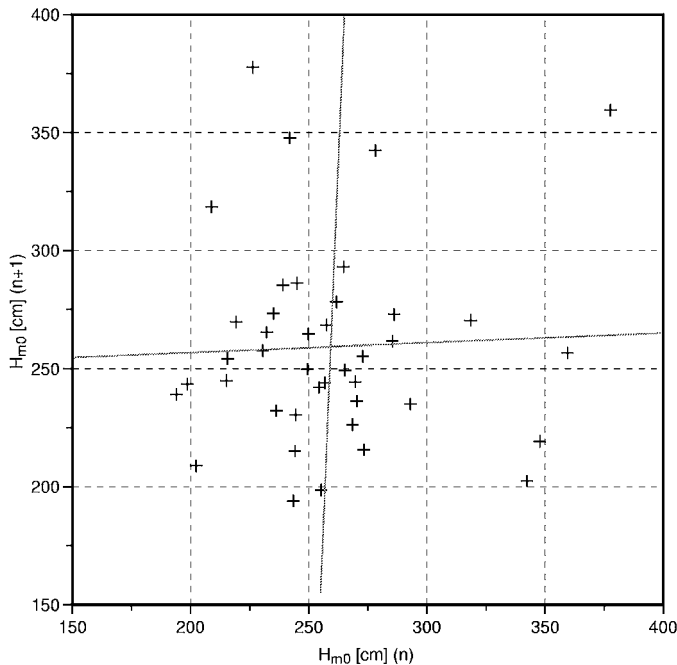
Abb. A 8.4: Korrelationsuntersuchungen von Extremwertdatensätzen, H_{m0,max} des Ereignisses n+1 als Funktion von H_{m0,max} des Ereignisses n mit zugehörigen linearen Regressionsgeraden, ( r = -0,02 ). Beispiel: Jahresmaxima signifikanter Wellenhöhen (FRÖHLE, 2000)
