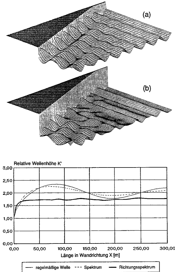
Abb. A 3.35: MACH-Reflexion von regelmäßigen Wellen und Spektren; oben: Wellenfeld vor einer senkrechten Wand bei regelmäßigem (a) und unregelmäßigem (b) Seegang (SCHEFFER, 1985); unten: Wellenhöhenverlauf in Wandrichtung für regelmäßige Wellen, eindimensionales Spektrum und Richtungsspektrum, Beispiel (DAEMRICH u. GÖTSCHENBERG, 1991)
