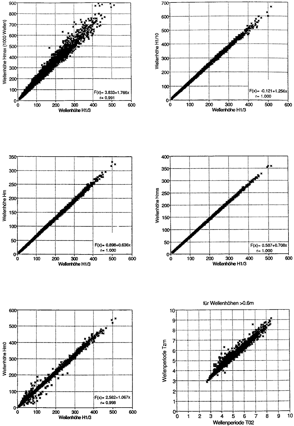
Abb. A 3.55: Kurzzeitstatistische Auswertungen von Seegangsmessungen, Beispiel Sylt (STROTMANN et al., 1992)
