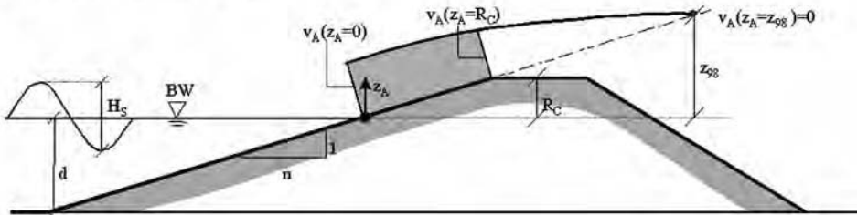
Abb. A 4.2.12: Definition der Strömungsparameter auf der Deichaußenböschung (SCHÜTTRUMPF, 2001)
