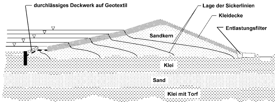
Abb. B 4: Schematische wasserstandsabhängige stationäre Sickerlinien im Deichkörper bei verschiedenen Sturmflutwasserständen
