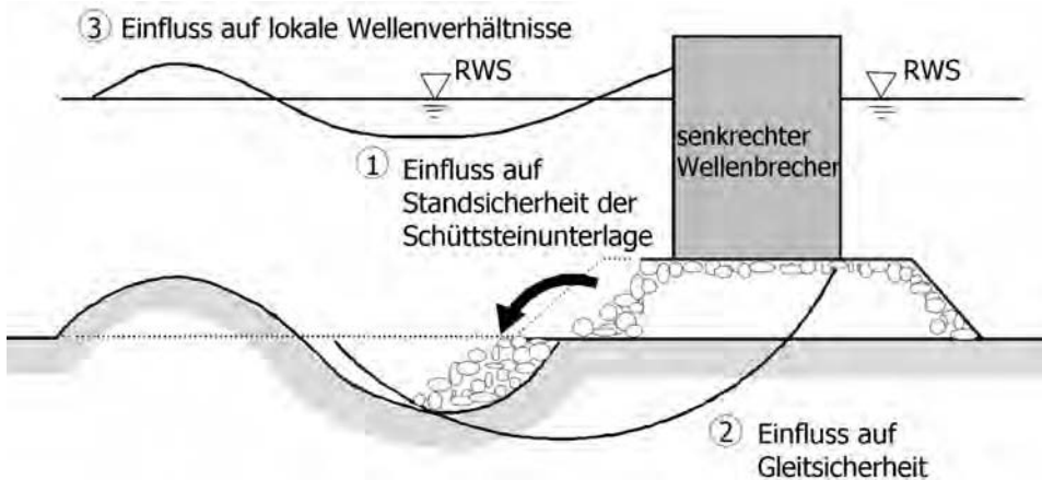
Abb. A 4.3.9: Einfluss der Kolkbildung auf die Standsicherheit der Schüttsteinunterlage und des Betonbauwerkes
