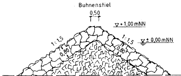
Schnitt A-A
