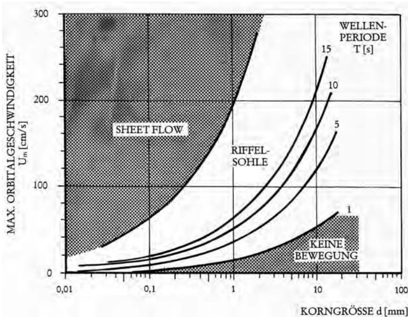
Abb. A 6.4: Schwellenwerte der Orbitalgeschwindigkeit an der Sohle u_m für Kornbewegungszustände und „Sheet-Flow“ von Quarzsand nach CLIFTON u. DINGLER (1984 in RAUDKIVI, 1990)
