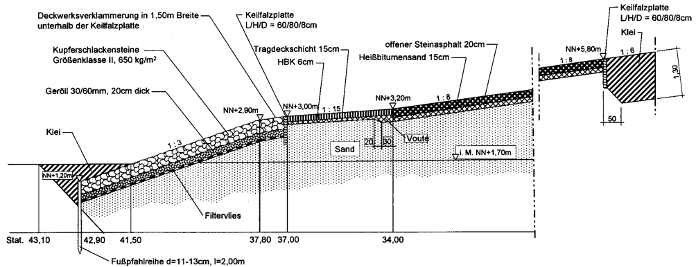
Abb. G 51a: Deichverstärkung Tümlauer Koog 1994/95: Deckwerk auf der Außenböschung auf 20 cm offenem Steinaspalt (Mastixschotter) auf 15 cm Bitumensand-Filter
