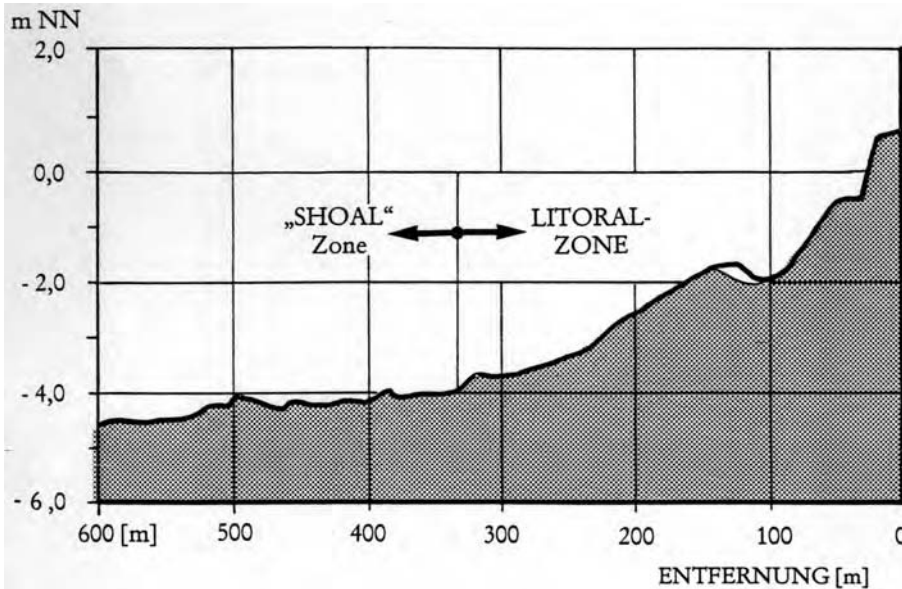
Abb. A 6.7: Veranschaulichung des Überganges von der Litoral- zur „Shoal“-Zone (Grenztiefe d_i ) am Beispiel eines Unterwasserstrandprofils der Ostsee
