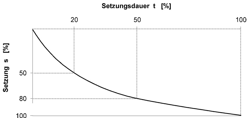
Abb. B 10: Typischer Zeit-Setzungsverlauf im Weichboden unter Deichneubauten
