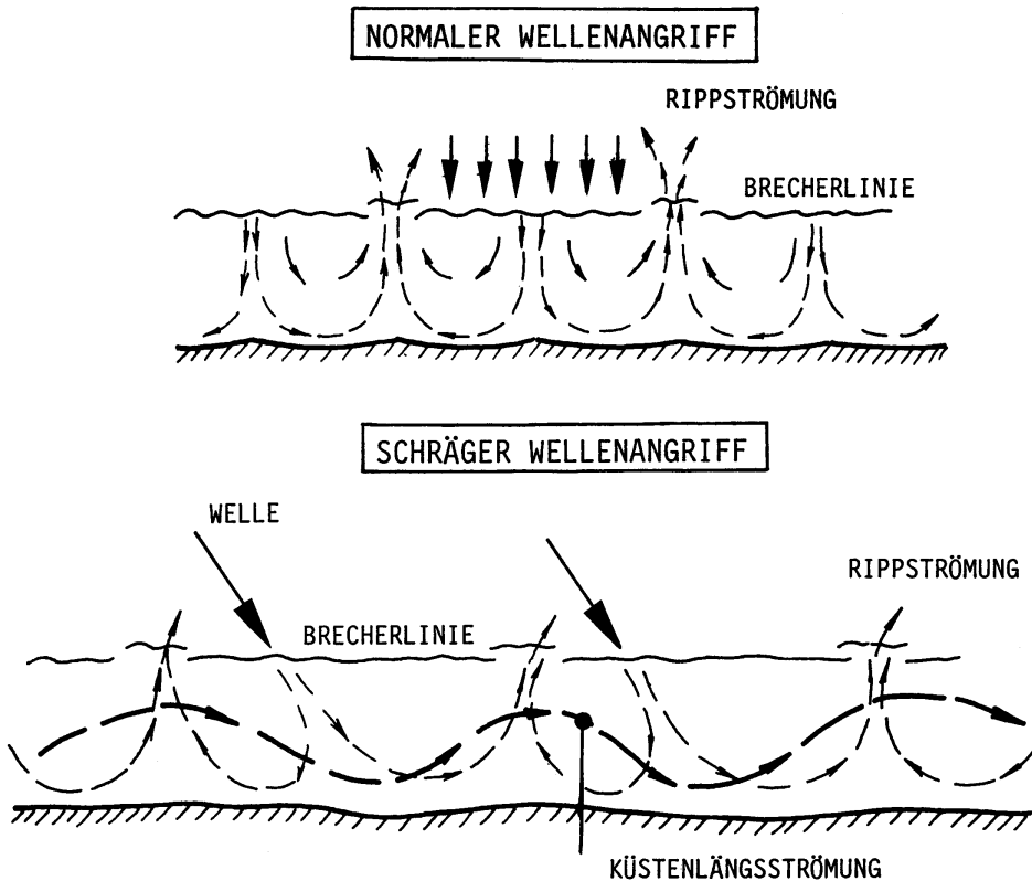
Abb. A 6.1: Ausbildung (schematisch) einer symmetrischen Zellenstruktur der Strömung sowie einer Rippströmung bei küstennormaler Wellenanlaufung (oben), mäandrierender Küstenlängsströmung sowie Rippströmung bei schräger Wellenanlaufung (unten).
