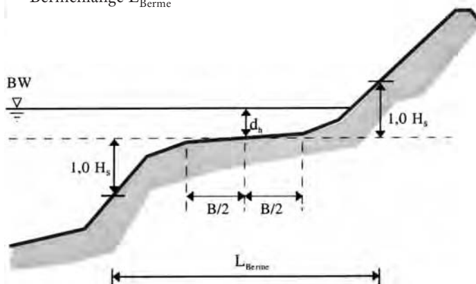
Abb. A 4.2.10: Berücksichtigung einer Berme im Deichquerschnitt bei der Ermittlung der Deichneigung \alpha und der wirksamen Bermenlänge L_{\text{Börmelänge}}
