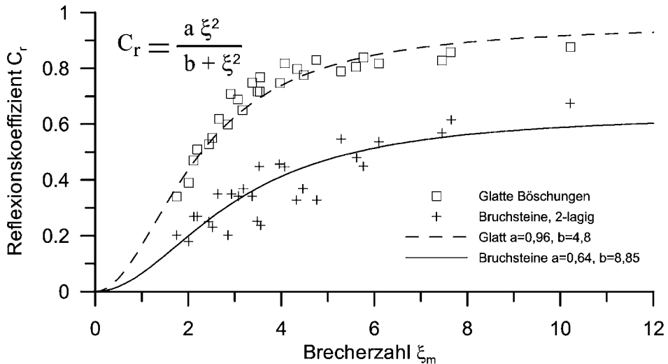
Abb. A 3.30: Reflexionskoeffizienten an glatten und rauen Schüttsteinböschungen (nach ALLSOP u. MCCONNEL, in HERBICH, 2000)
