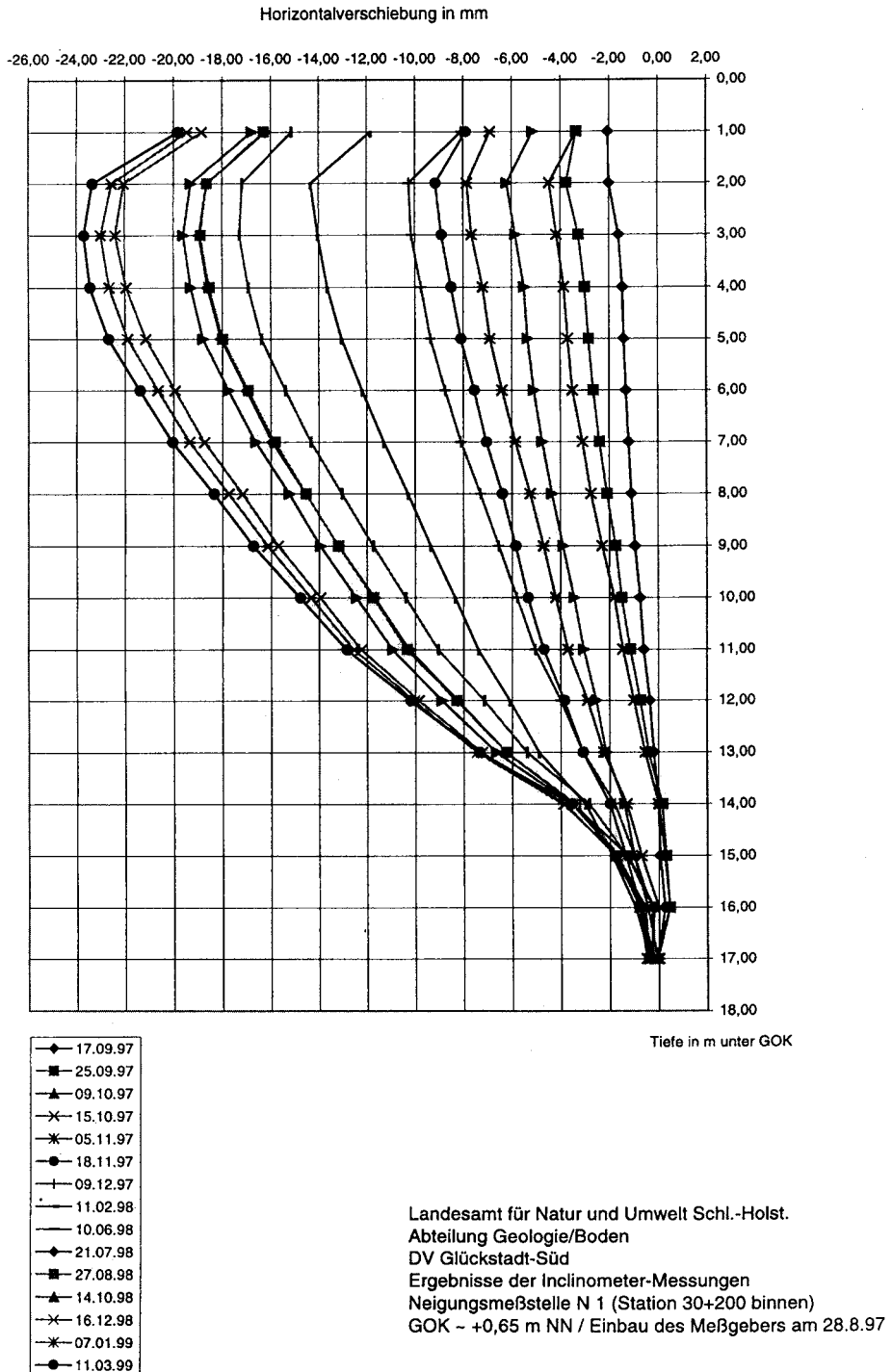
Abb. B 17: Tiefenbezogene Darstellung der Horizontalverschiebungen bei Dkm 30 + 200 Glückstadt-Süd
