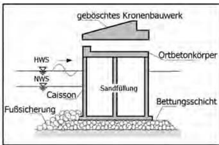
(a) senkrechter Wellenbrecher
