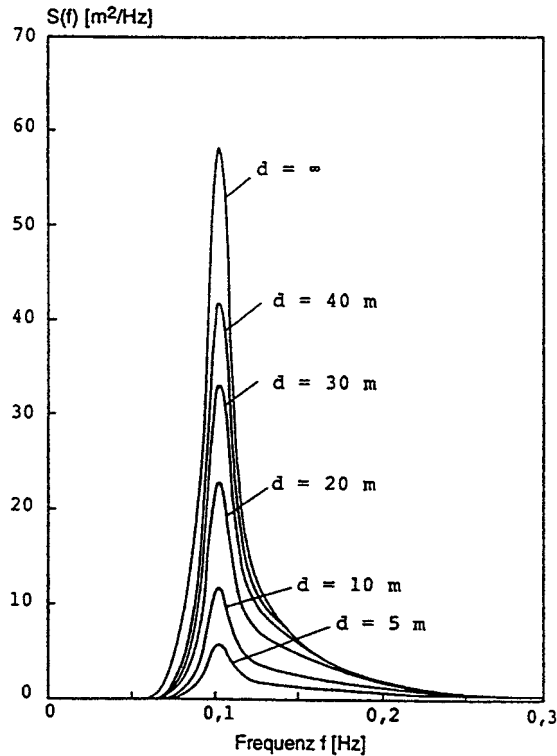
Abb. A 3.15: TMA-Flachwasserspektrum für unterschiedliche Wassertiefen, bei sonst gleichen Parametern f_p , \alpha , \gamma , \sigma_a und \sigma_b (SCHADE, 1991)
