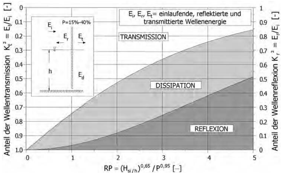
Abb. A 4.3.6: Funktionskurven einer einfachen vertikalen durchlässigen Wand (ohne Wellenkammer)
