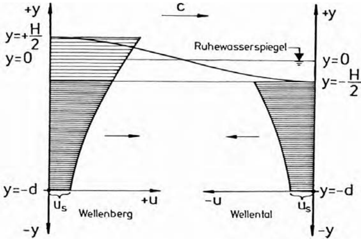
Abb. A 5.8. Schematische Darstellung der Abnahme der Horizontalkomponenten der Orbitalgeschwindigkeiten mit der Wassertiefe
