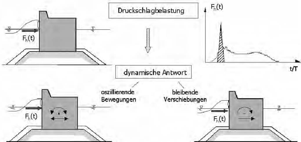
Abb. A 4.3.5: Einfluss der Druckschlagbelastung auf das Gesamtbauwerk
