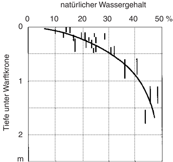
Abb. B 11: Zunahme des Wassergehaltes mit der Tiefe in bindigen Abdeckböden von Warftverstärkungen auf der Hallig Langeness (gemessen am 15.5.1996, TEMMLER LANU SH)
