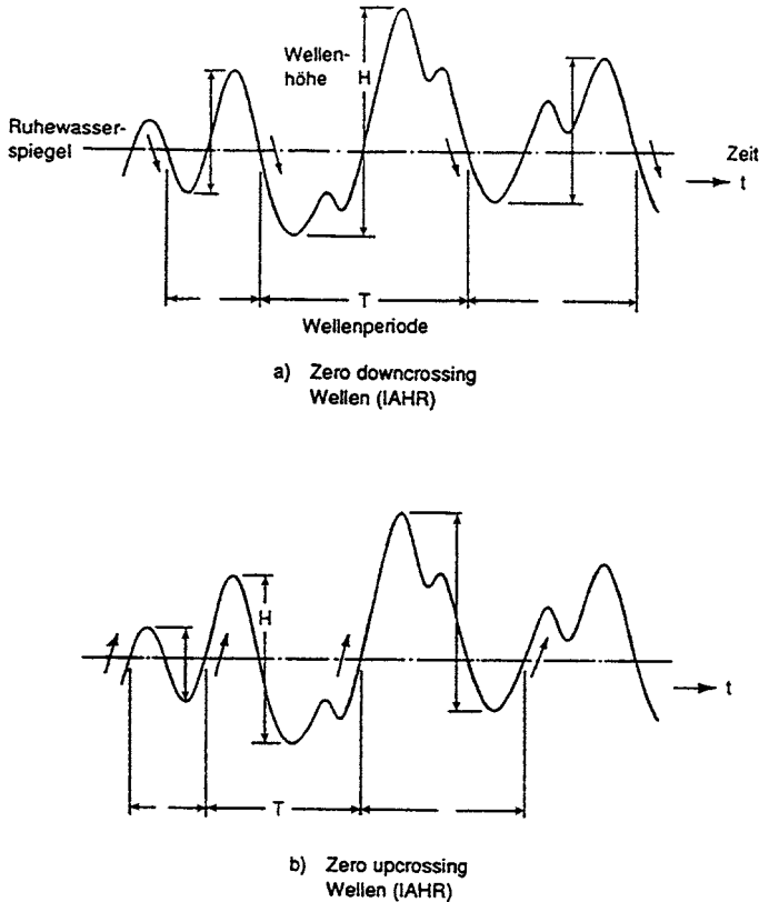
Abb. A 3.10: Zur Definition von zero crossing Wellenhöhen (nach IAHR/PIANC, 1986)
