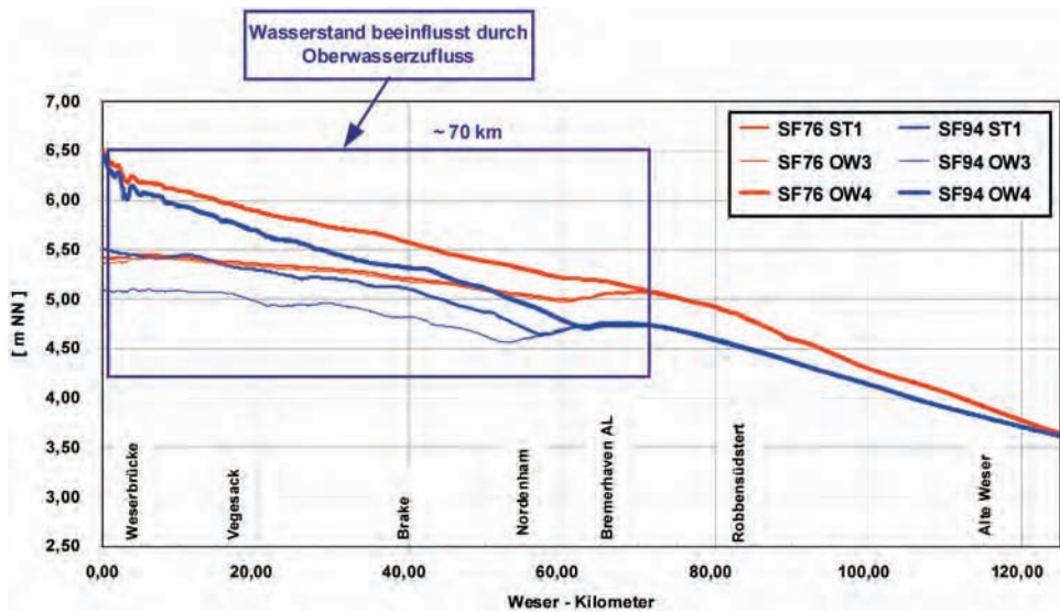
Abb. A 2.5: Sturmflutscheitelwasserstände der Weser (Sturmflut vom 3. Jan. 1976); siehe auch Tab. A 2.1
