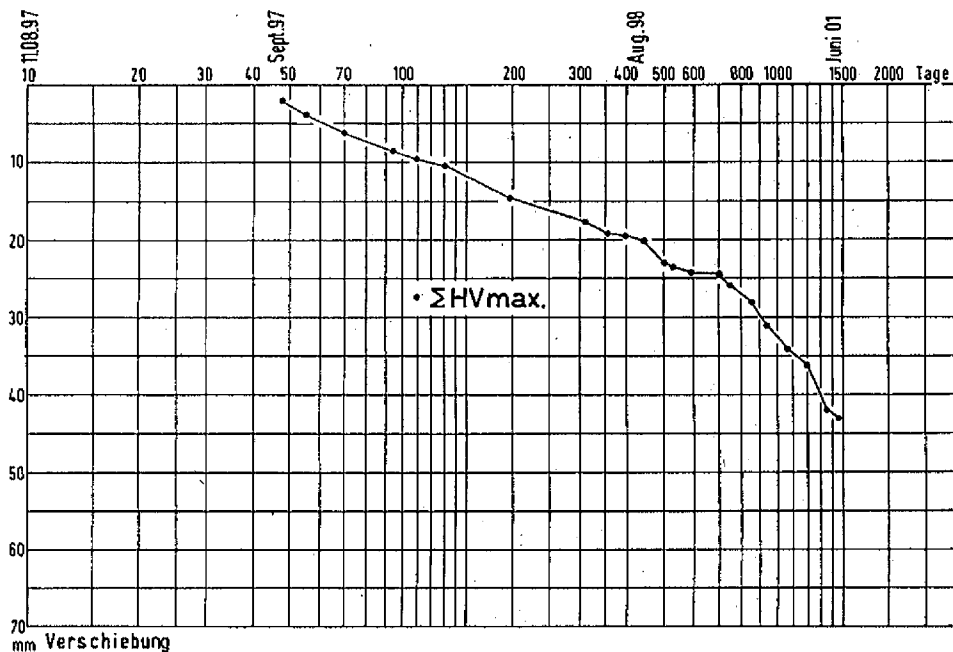
Abb. B 18: Zeitliche Veränderung der maximalen Hauptverschiebung bei DKm 30 + 200 Glückstadt-Süd
