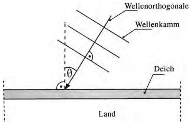
Abb. A 4.2.11: Definition des Wellenangriffswinkels \theta
