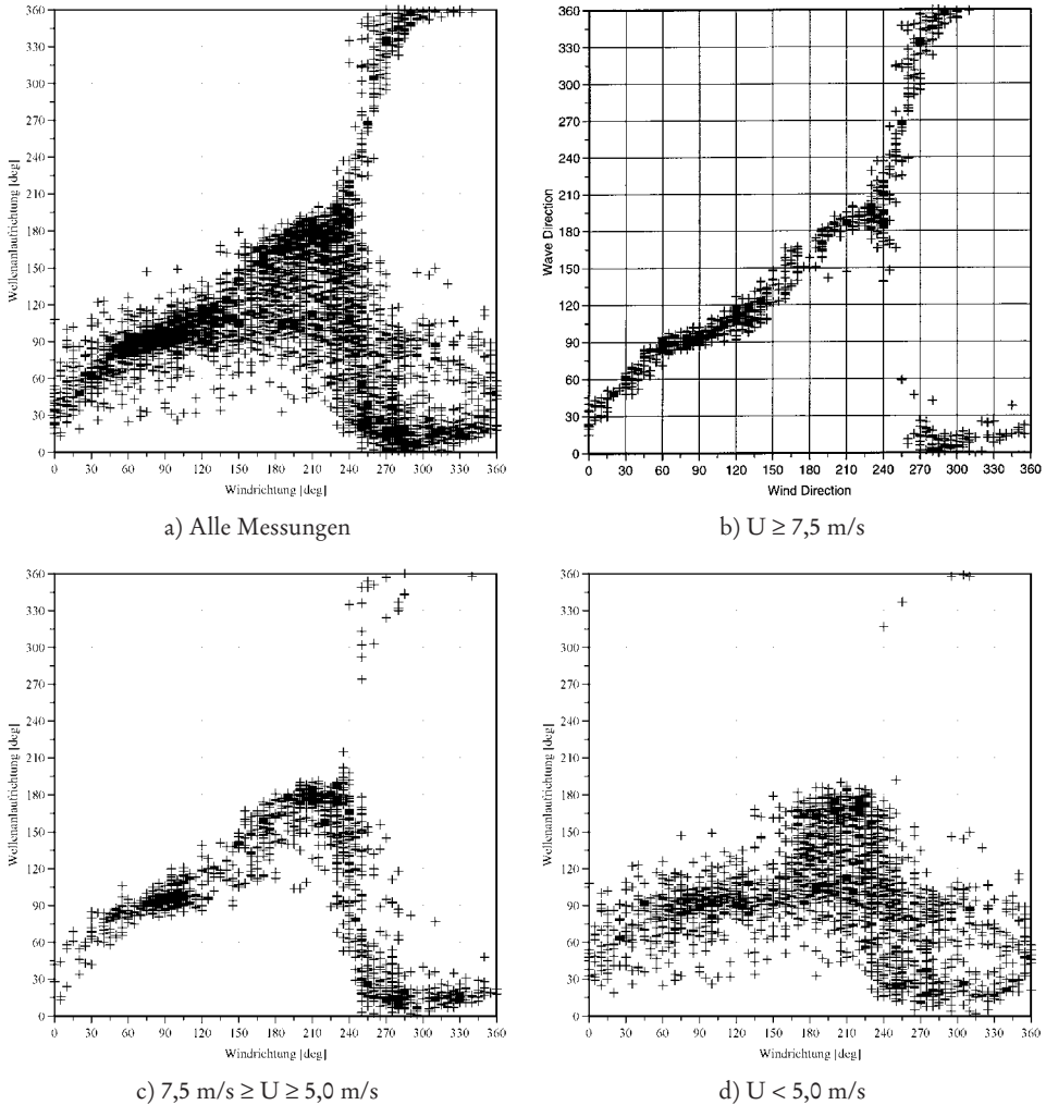
Abb. A 3.48: Gemessene Wind- und Wellenrichtungen (Projektgebiet Schönhagen, FRÖHLE et al., 1999)
