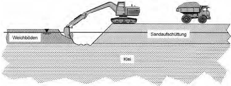
Abb. G 37: Räumung des Weichbodens durch Tieföffelbagger
