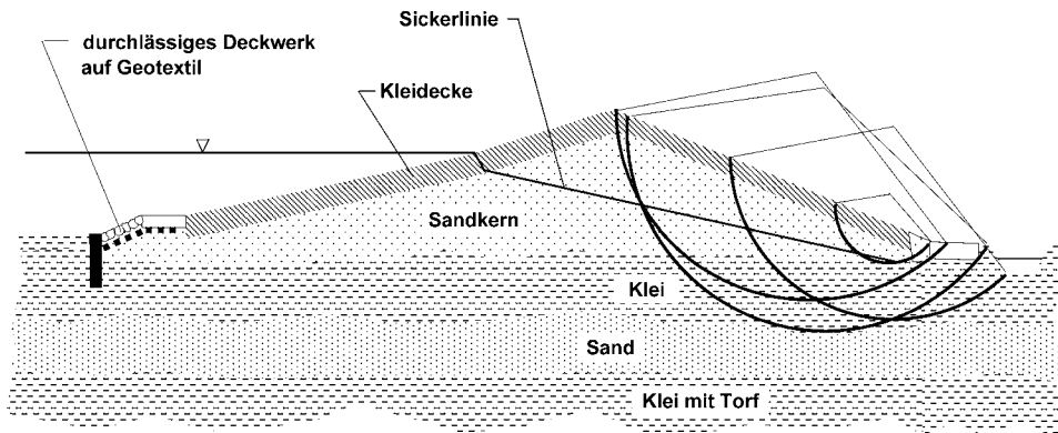
Abb. B 5: Nachweis der globalen Standsicherheit an der luftseitigen Böschung
