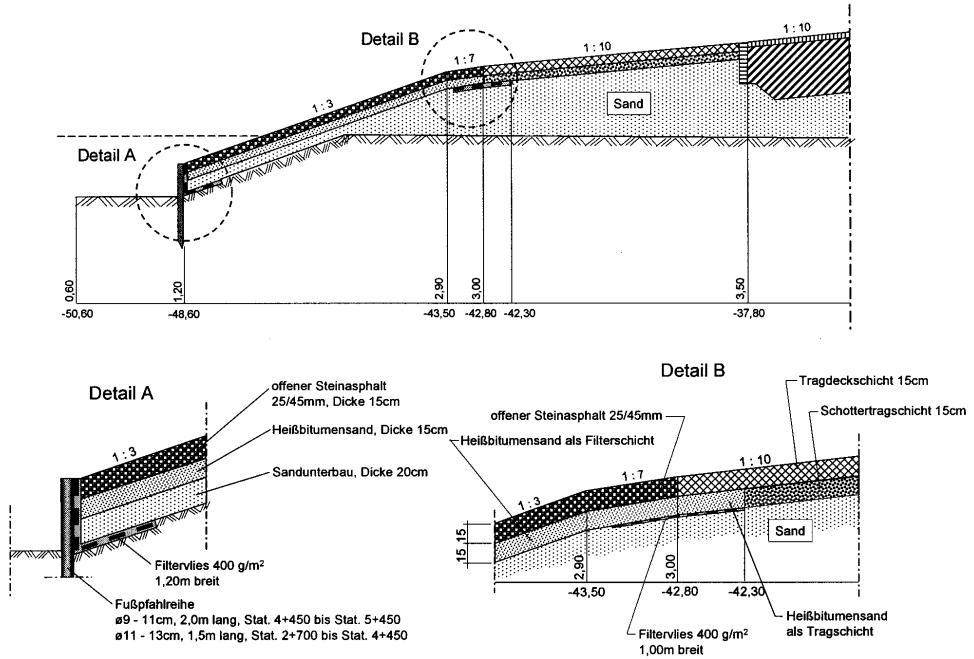
Abb. G 50a: Deichverstärkung Friedrich-Wilhelm-Lübke-Koog hinter Vorland 2001/2002 aus 15 cm Mastixschotter auf 15 cm Bitumensand-Filter bis zur Überschlagssicherung
