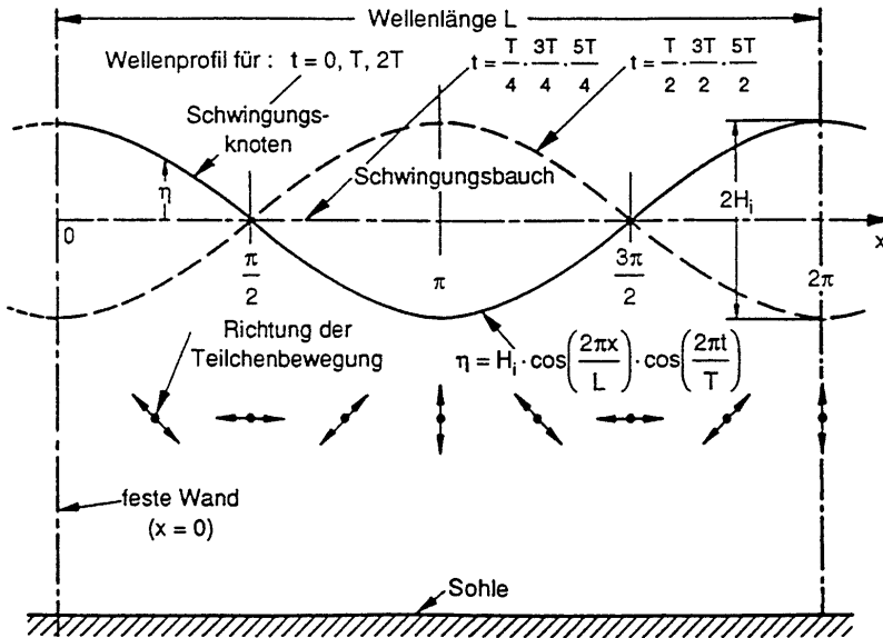
Abb. A 3.28: Stehende Welle an einer senkrechten Wand (Clapotis), nach CERC (1977)
