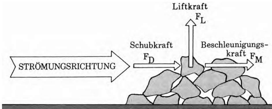
Abb. A 5.10: Belastung eines Einzelsteins eines Deckwerkes infolge Überströmung
