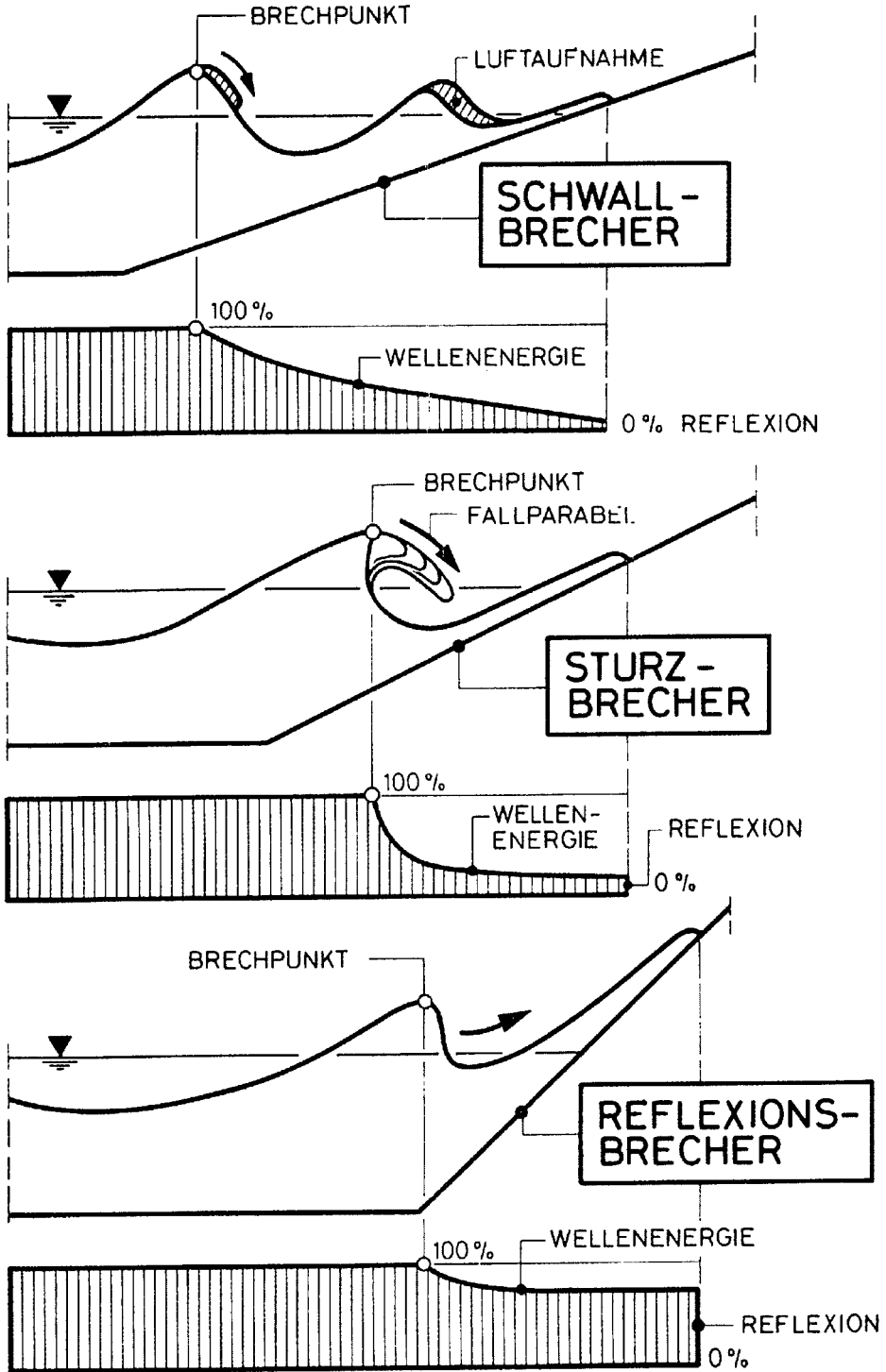
Abb. A 4.2.2: Brecherformen (schematisch) (aus FÜHRBÖTER, 1991)
