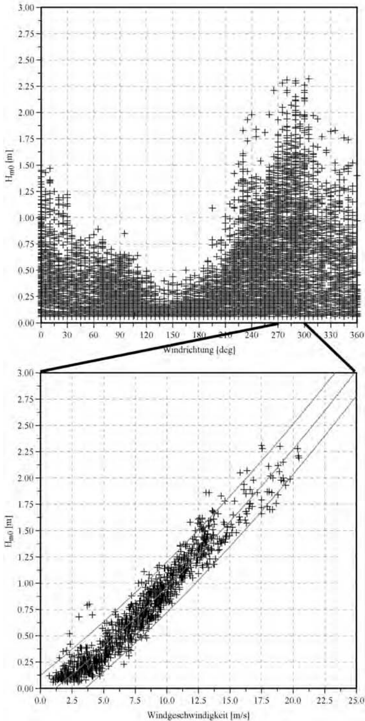
Abb. A 3.47: Gemessene signifikante Wellenhöhen in Abhängigkeit von der mittleren Windgeschwindigkeit im Projektgebiet Heiligenhafen und Korrelationsfunktion mit zugehörigem 90 % Konfidenzintervall. Beispiel Windrichtungsklasse 270^\circ \leq \Theta_{\text{wind}} < 300^\circ (FRÖHLE u. FITTSCHEN, 1999)
