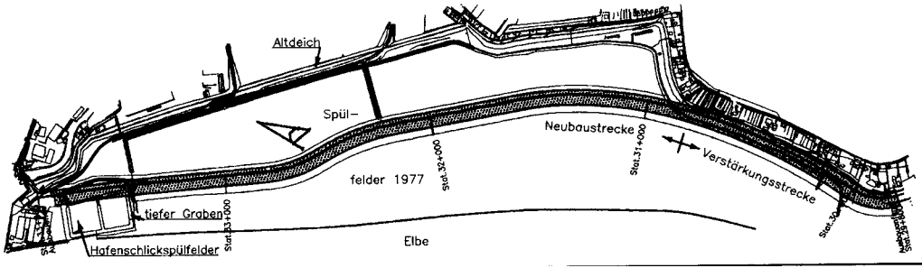
Abb. B 12: Lageplan der Deichbaumaßnahme
