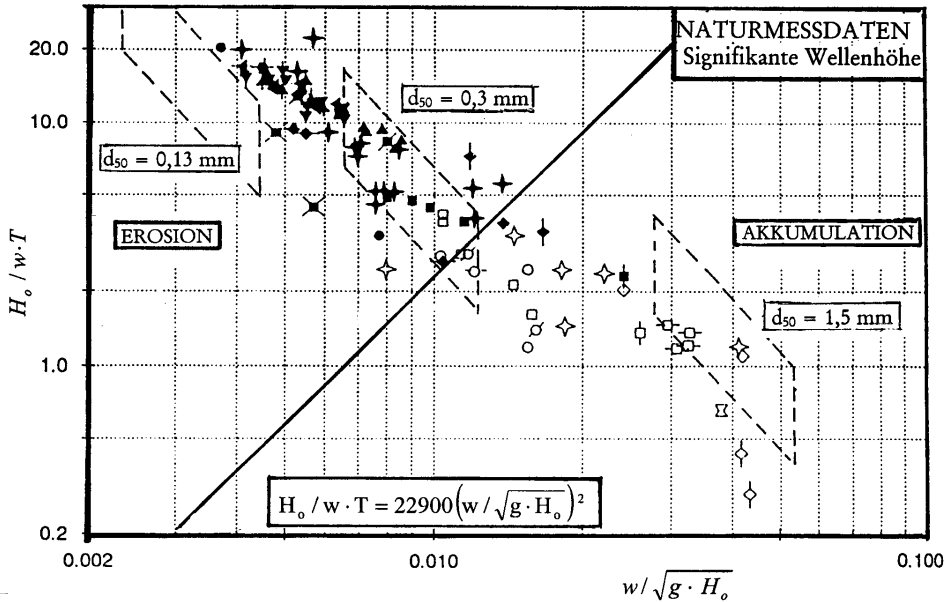
Abb. A 6.3: Kriterien für Erosion und Akkumulation; hier Darstellung von Naturmessdaten als H_{0s}/w \cdot T in Abhängigkeit von w/(g \cdot H_{0s})^{1/2} . Die Bereiche, begrenzt durch 4 \leq T \leq 10 s; 0,5 \leq H_{0s} \leq 2,0 m sind für Korngrößen 0,13 mm, 0,3 mm und 1,5 mm zur Veranschaulichung eingezeichnet (KRAUS et al., 1991).
