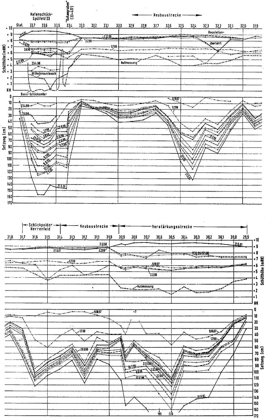
Abb. B 14: Schütthöhen und Setzungen entlang der Deichtrasse Glückstadt-Süd
