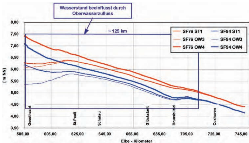
Abb. A 2.6: Sturmflutscheitelwasserstände der Elbe (Sturmflut vom 24. Jan. 1994); siehe auch Tab. A 2.1
