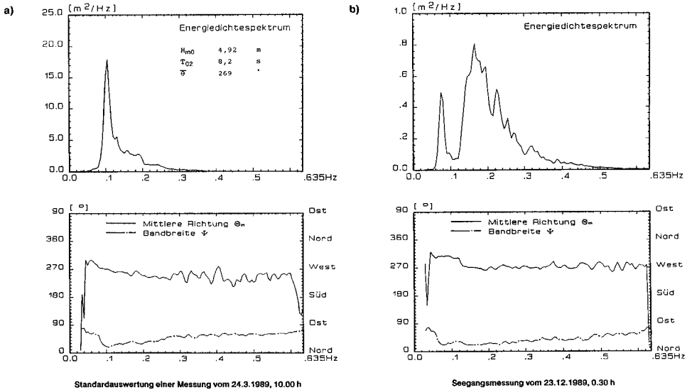
Abb. A 3.45: Zur Auswertung von Richtungsspektren, Beispiel Sylt, WAVEC-Messungen (SCHADE, 1991)
