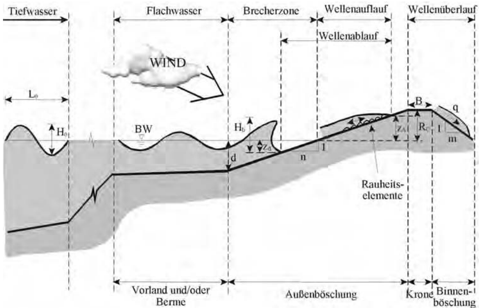
Abb. A 4.2.7: Schematische Darstellung des Wellenauflaufes (SCHÜTTRUMPF, 2001)
