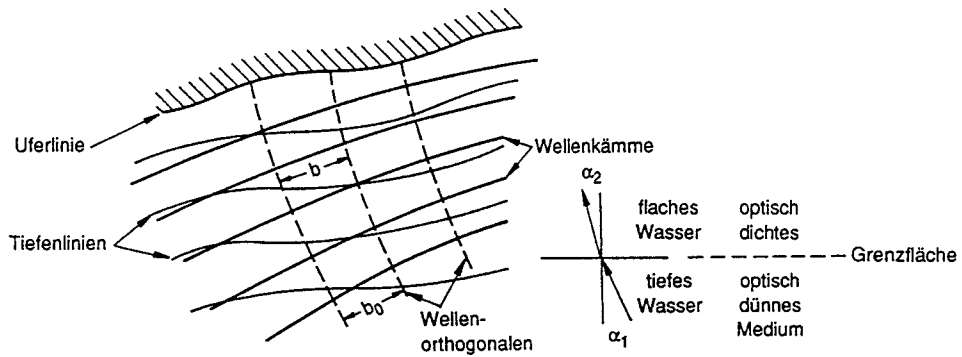
SNELLSche Analogie
