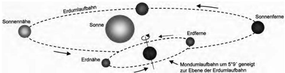
Abb. A 5.3: Erde-Mond-Sonne-System
