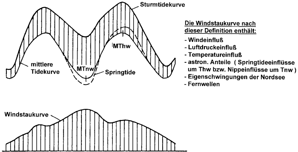
Abb. A 2.7: Windstaukurve als Differenz zwischen der eingetretenen und der vorausberechneten astronomischen oder der für diese Zeit gebildeten mittleren Tide (SIEFERT, 1998)
