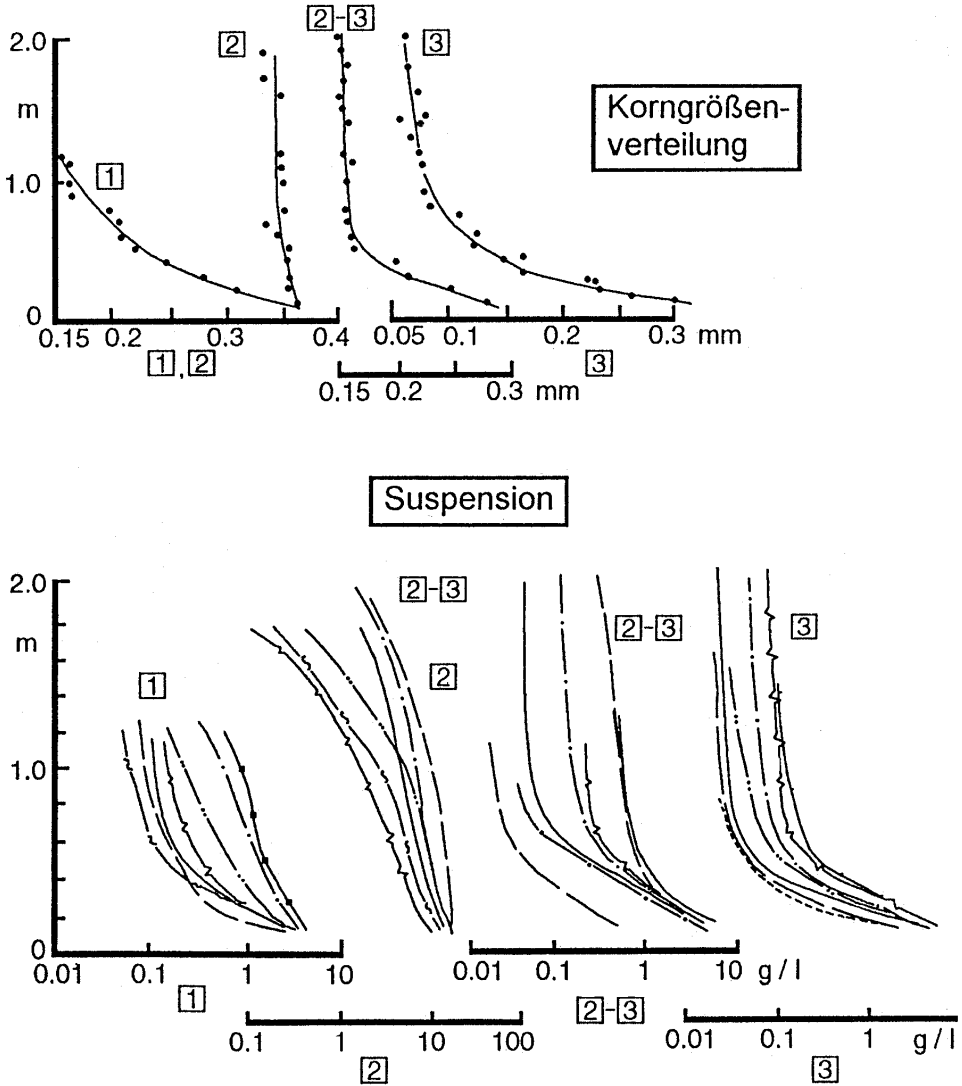
Abb. A 6.10: Korngrößen- und Konzentrationsverteilungen des suspendierten Sedimentes an vier Stationen entlang eines Querprofils am Schwarzen Meer (KOS'YAN et al., 1982 nach EAK, 1993)
