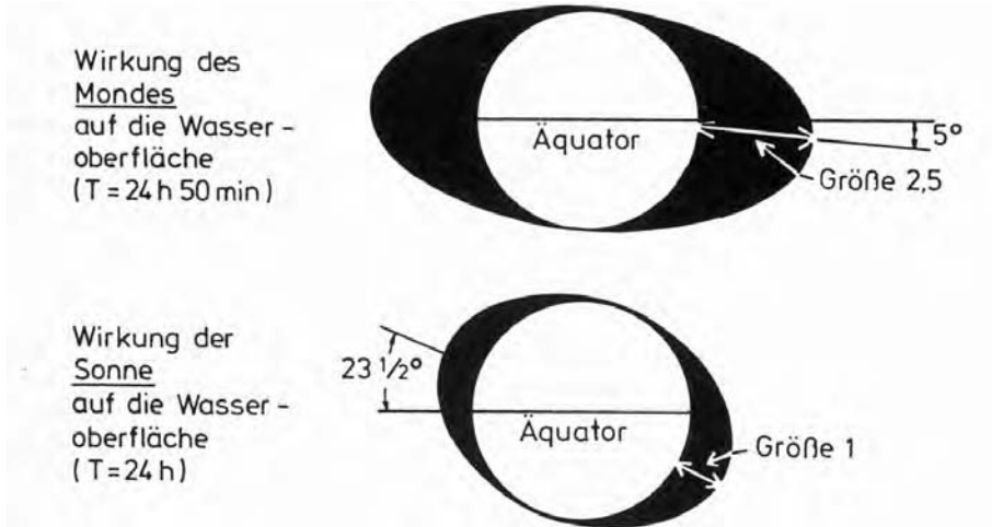
Abb. A 5.2: Wirkungen des Mondes und der Sonne auf die Wasseroberfläche
