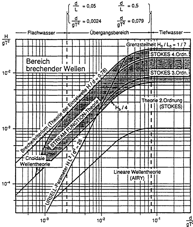
Abb. A 3.5: Anwendungsbereiche verschiedener Wellentheorien (nach CERC, 1984)
