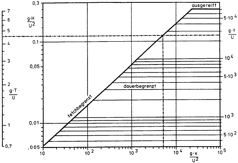
Abb. A 3.39: Dimensionslose Darstellung von fetch- und dauerbegrenztem Windseegang (RICHTER, 1979)
