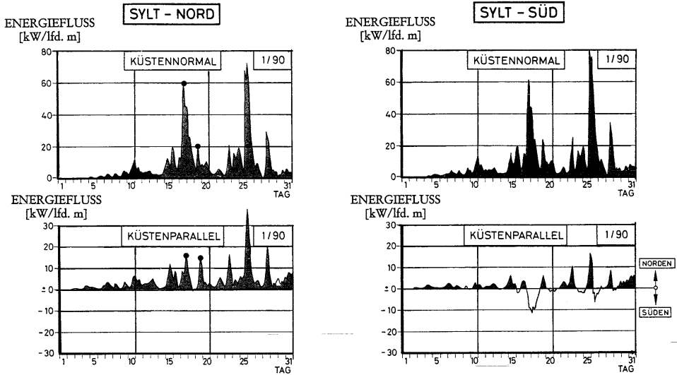
Abb. A 6.12: Zeitreihe der Komponenten (küstennormal und küstenparallel) des resultierenden Energieflusses in die Brandungszonen von Sylt-Süd und Sylt-Nord im Januar 1990 (DETTE, 1991)
