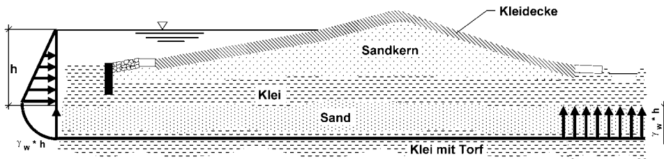
Abb. B 8: Hydraulischer Grundbruch landseitig vom Deichfuß
