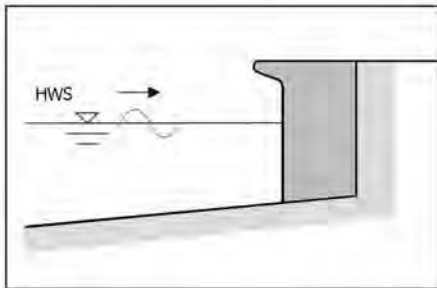
(c) Strand- und Ufermauer
