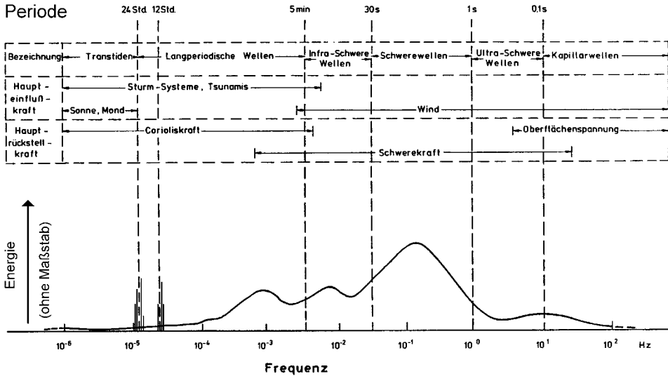
Abb. A 3.1: Einteilung ozeanischer Oberflächenwellen mit einer Einschätzung des relativen Energieinhalts (CERC, 1977)
