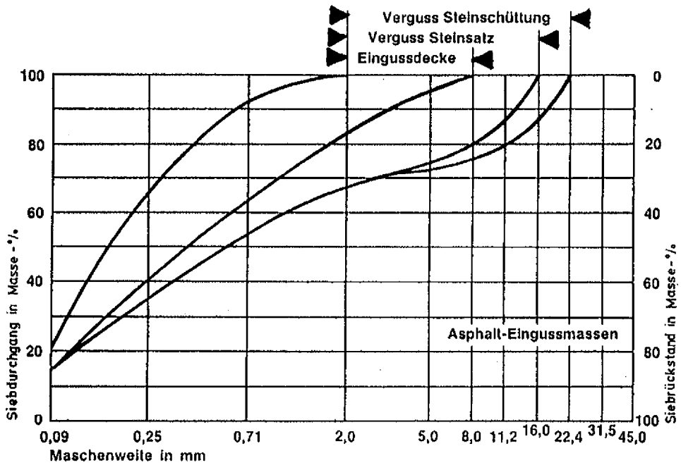
Abb. C 4: Sieblinienbereich für Asphalt-Eingussmassen (Asphaltmastix), (EAAW 83/96)
