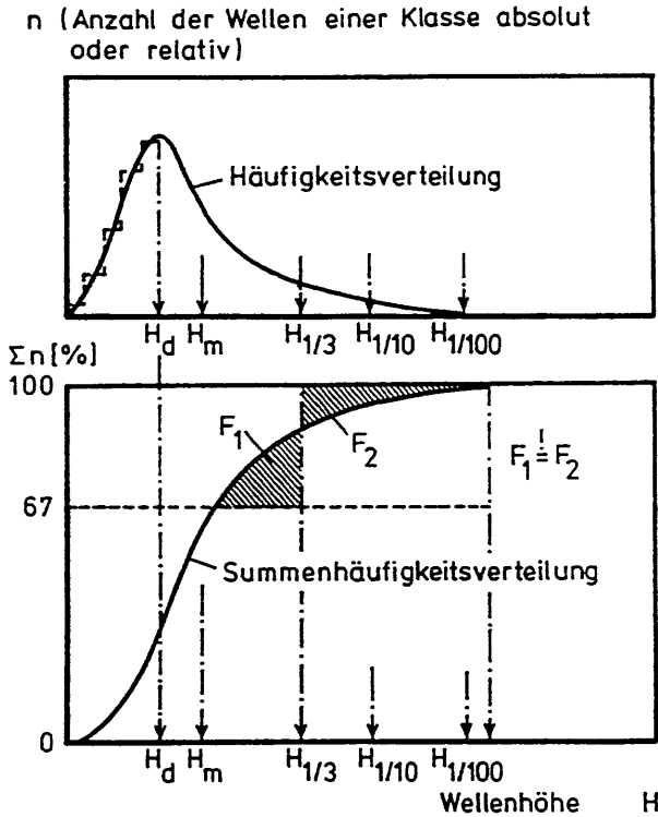
Abb. A 3.11: Prinzip der Auswertung von Zeitbereichparametern aus einer Häufigkeitsdarstellung (Histogramm) ( H_d ist hier die „dominante“ Welle und nicht zu verwechseln mit dem im Folgenden verwendeten Index d für downcrossing)
