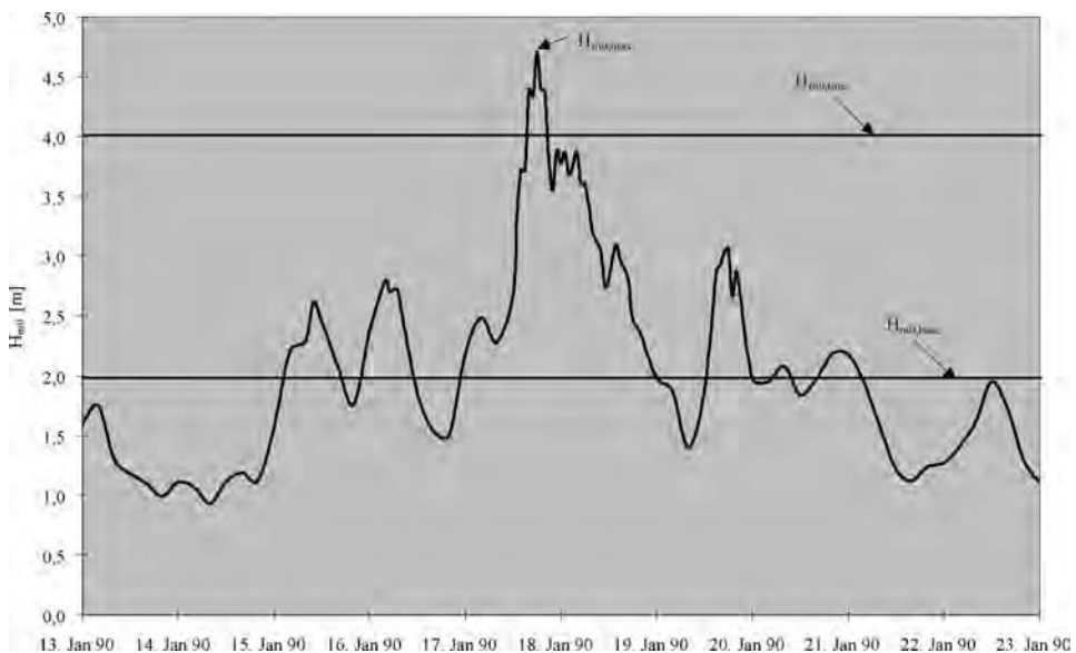
Abb. A 8.3: Zur Definition von Peak-Over-Threshold-Werten (POT-Werten)
