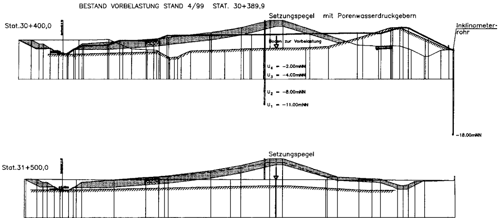
Abb. B 13: Charakteristische Deichquerschnitte
