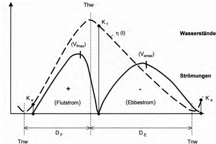
Abb. A 5.5: Parameter zur Beschreibung der Tide
