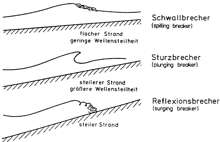
Abb. A 3.21: Klassifizierung der Brecherformen, schematisch
