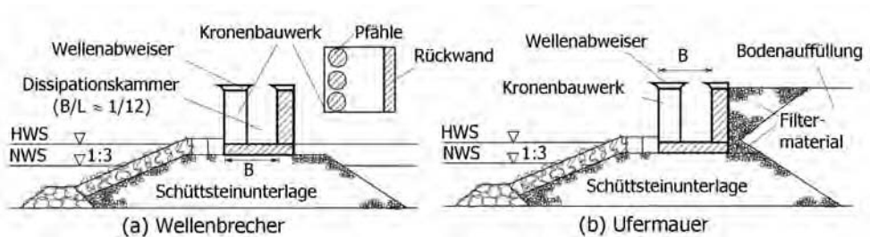
Abb. A 4.3.8: HMCB-Konzept mit Dissipationskammer als Wellenbrecher bzw. Ufermauer
