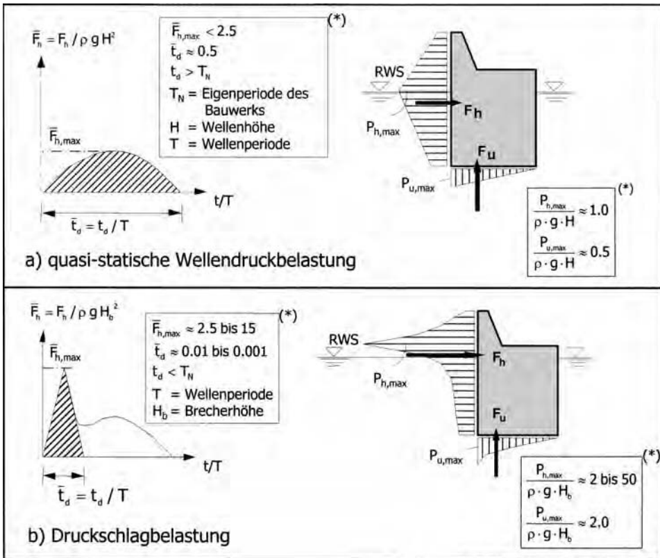
Abb. A 4.3.4: Unterschied zwischen quasi-statischer und Druckschlagbelastung
