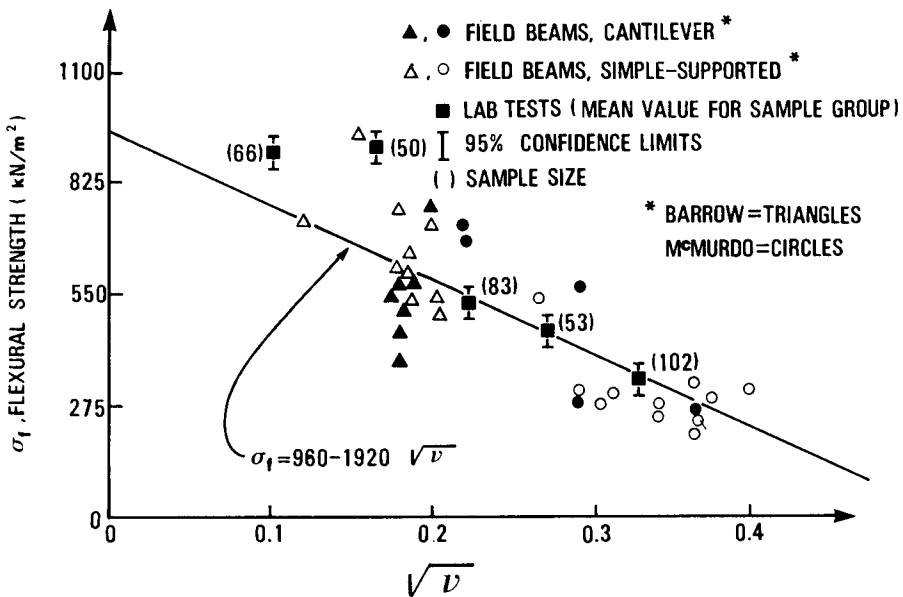
Abb. A 7.9: Biegefestigkeit von Meer-Eis als Funktion des Salzlaugenvolumens (nach VAUDREY, 1977)
