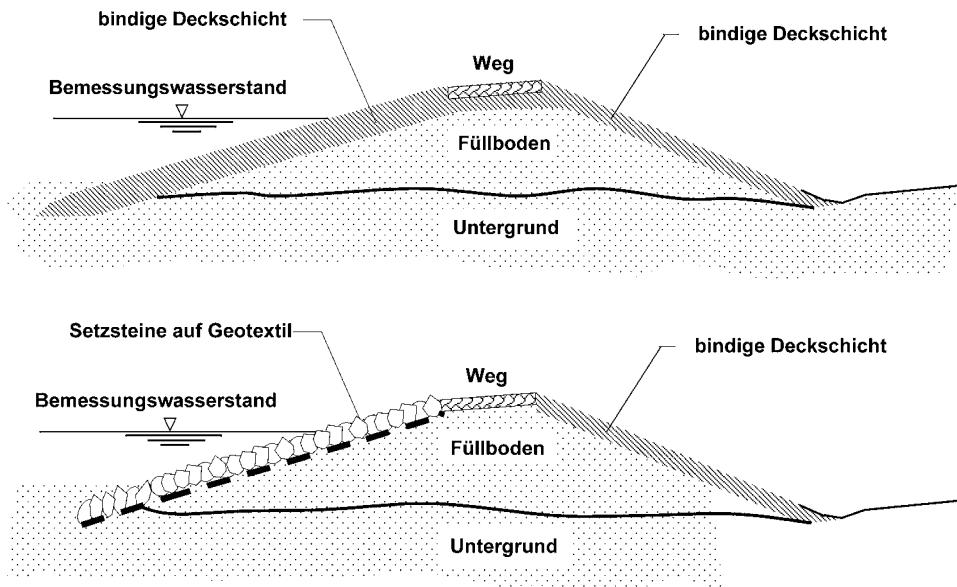
Abb. B 2: Bodenaufbau von Deichprofilen an der Ostseeküste
