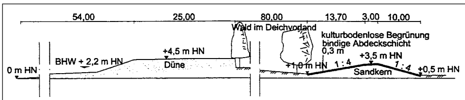
Abb. G 2: Seedeich Ückeritz (Schmollenseeniederung), Mecklenburg-Vorpommern
