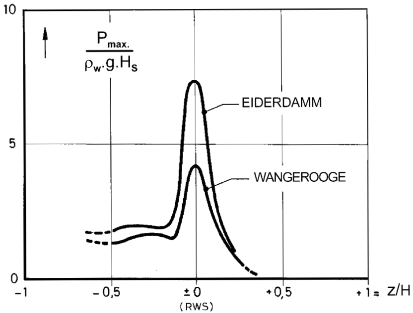
Abb. A 4.2.5: Naturuntersuchungen von GRÜNE (1988) mit Böschungsneigungen 1:n = 1:4: Druck-schlaghöhen und -bereiche bei natürlichen Wellenspektren (aus FÜHRBÖTER, 1991)
