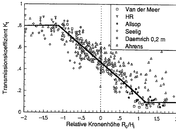
Abb. A 3.36: Wellentransmission an Schüttsteinwellenbrechern mit niedriger Kronehöhe (VAN DER MEER u. D'ANGREMOND, 1991)
