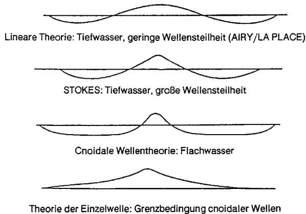
Abb. A 3.4: Zur Anwendung von Wellentheorien (aus LE MEHAUTE, 1976) oben: Teilchenbewegung in oszillatorischen und translatorischen Wellen, schematisch unten: Verdeutlichung unterschiedlicher Wellenprofile bei Verwendung verschiedener Theorien
