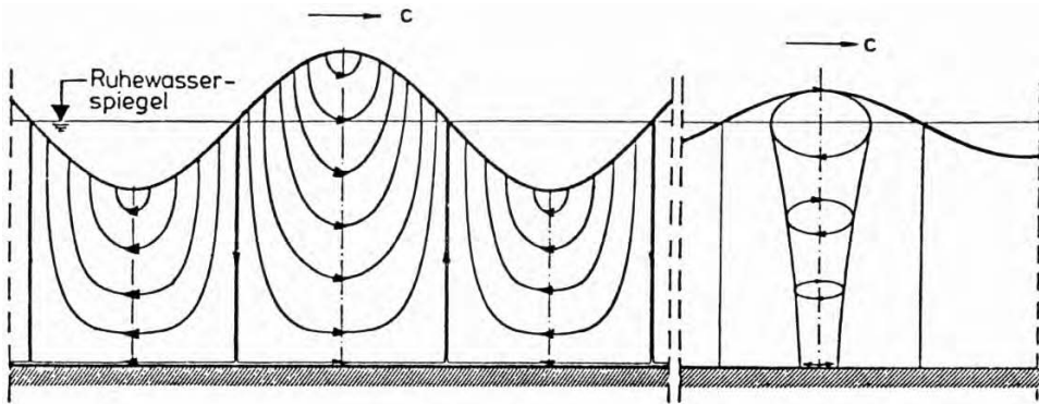
Abb. A 5.7: Stromlinien (links) und Orbitalbahnen (rechts) unter einer fortschreitenden Welle mit Grundberührung
