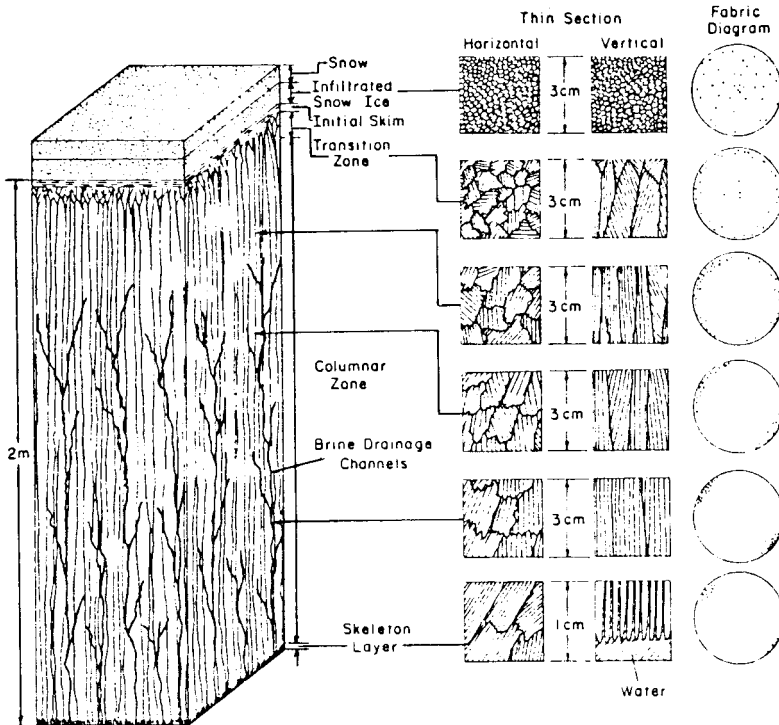
Abb. A 7.3: Schematische Darstellung mit den verschiedenen Schichten von einjährigem Meer-Eis (nach SCHWARZ u. WEEKS, 1977)
