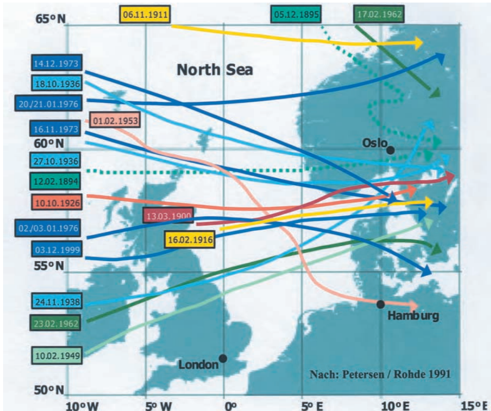
Abb. A 2.3: Zugbahn der Nordsee-Orkantiefs (nach PETERSEN u. ROHDE, 1991)
