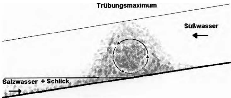
Abb. A 5.6: Salzkeileffekt (nach WELLERSHAUS, 1982)
