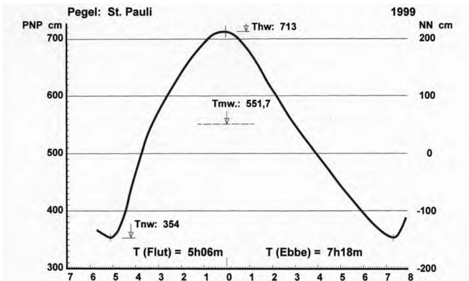
Abb. A 5.4: mittlere Tidekurve am Pegel St. Pauli
