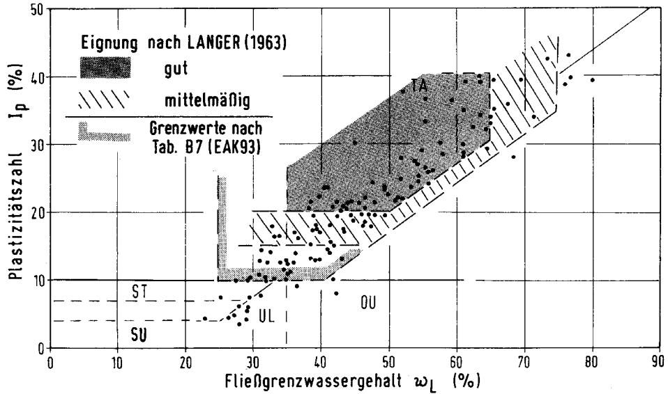
Abb. G 23: Plastizitätskarte von Deichabdeckböden an der Nordseeküste
