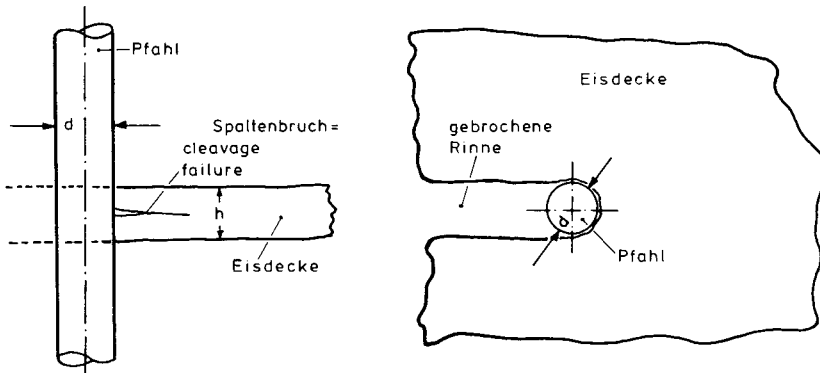
Abb. A 7.11: Spaltbruchversagen der Eisdecke
