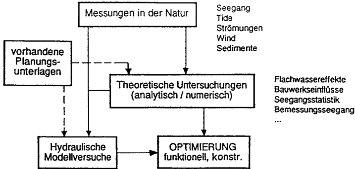
Abb. A 3.2: Untersuchung von Seegangsproblemen im Küstenwasserbau, methodische Wechselbeziehungen
