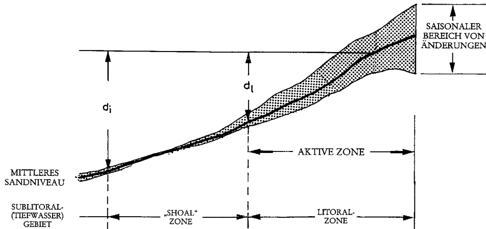
Abb. A 6.6: Aufteilung des Unterwasserprofils im Küstenvorfeld auf der Grundlage von Grenziefen („closure depths“), hier: d_1 als Grenze, bis zu der sich jahreszeitliche oder saisonale Änderungen des Ober- und Unterwasserstrandprofils in beachtlichen Größenordnungen abspielen und d_i als Grenze, wo das mittlere jährliche Wellenklima noch eine Sedimentbewegung bewirkt (HALLERMEIER, 1981)
